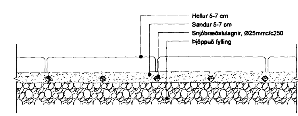
KENNISNIÐ SNJÓBRÆÐSLU Í HELLUR 1:10
