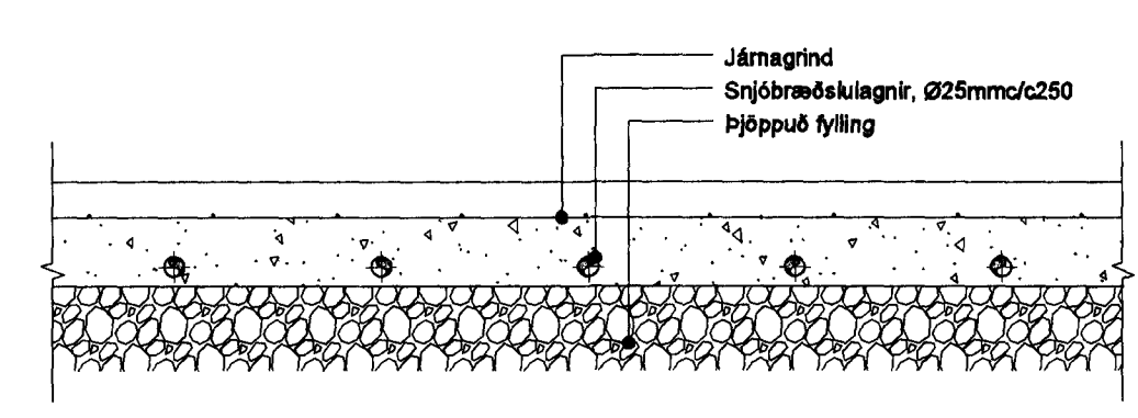
KENNISNIÐ SNJÓBRÆÐSLU Í PLAN 1:10
