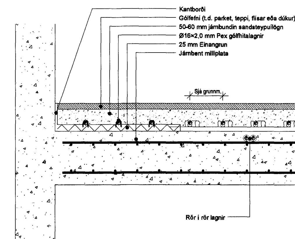
KENNISNIÐ GÓLFHITA 1:10
