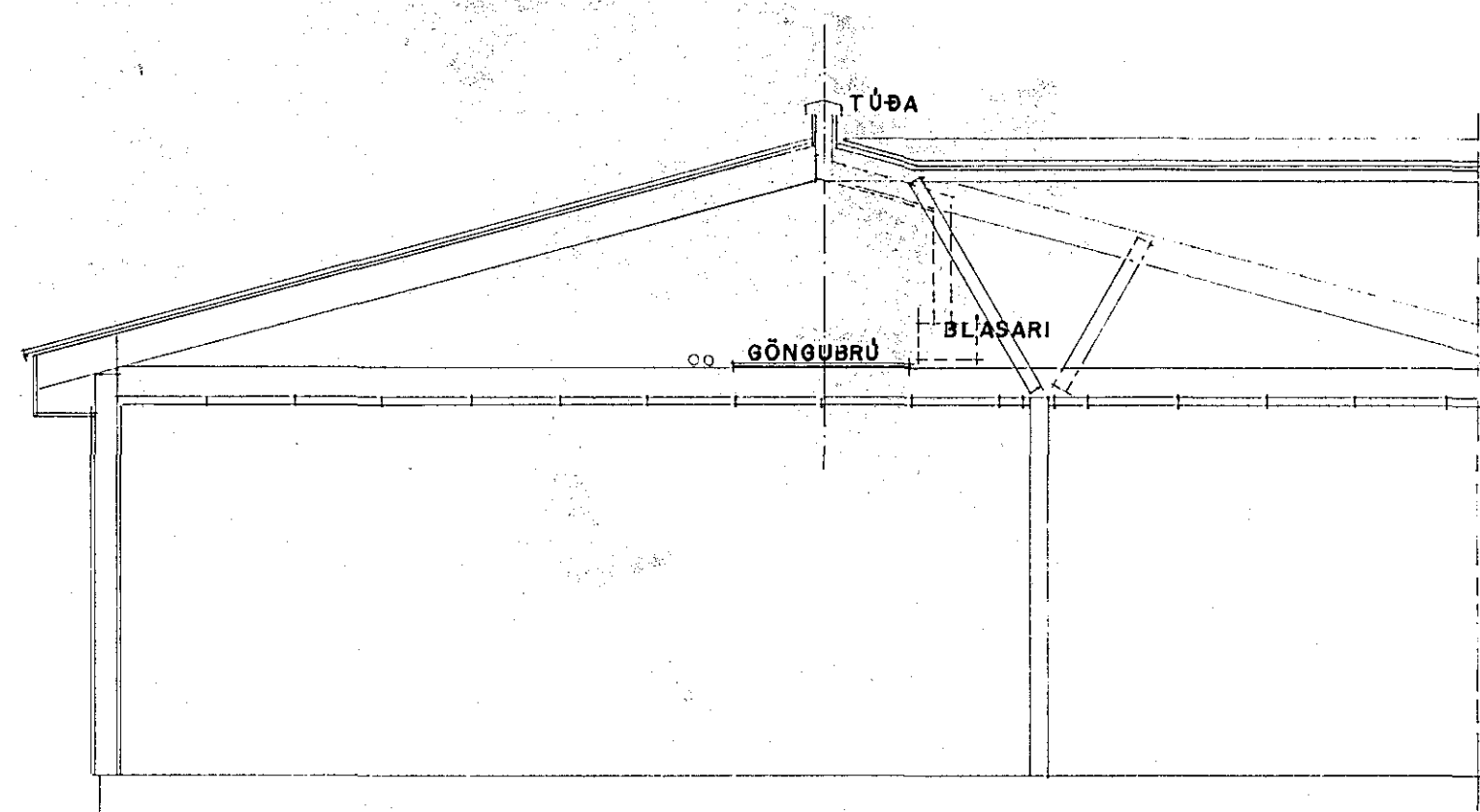
SNEIDING 1:50
