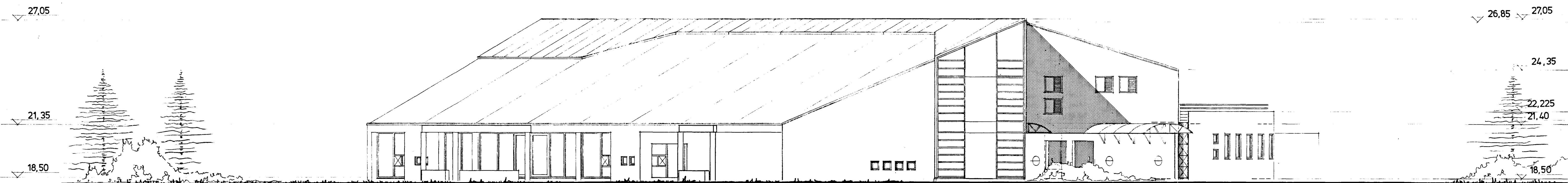
SUÐ-AUSTURGAFL
