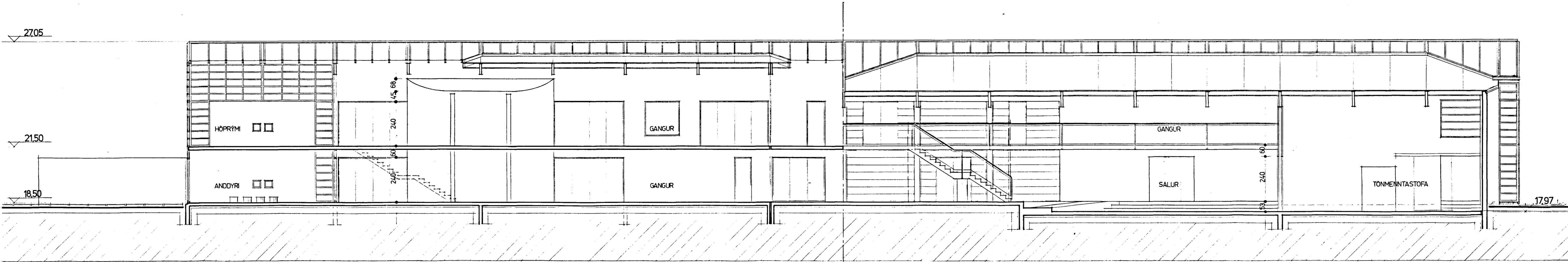
SNEIDING C-C
