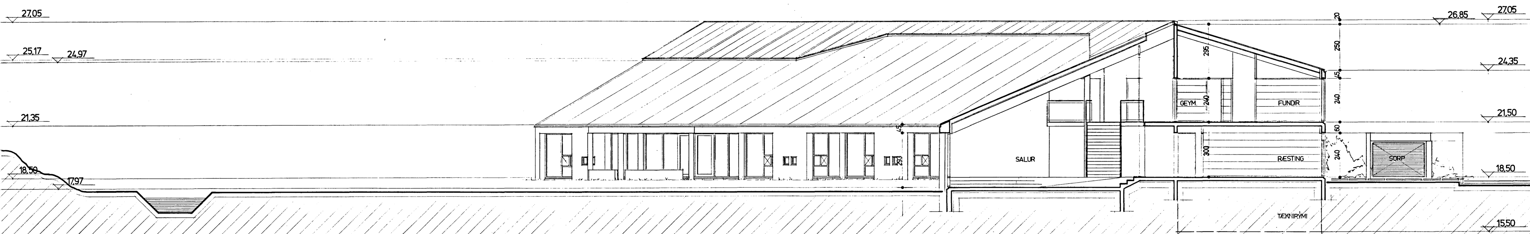
SNEIDING B-B
