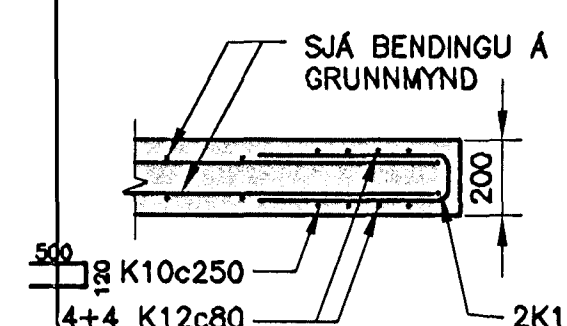
D07 LÓDRÉTT SNID - FRÁGANGUR Á PLÖTUBRÓN MKV. 1
