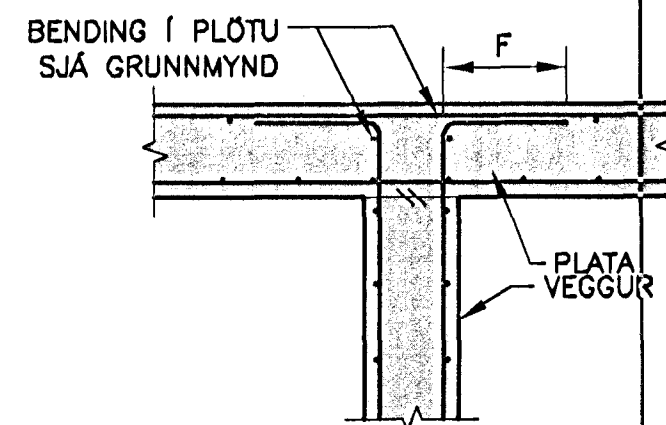
D02 DÆMIGERD JÁRNBENDING Í SAMSKEYTUM VEGGJA OG PLATNA - LÓDRÉTT SNID MKV. 1
