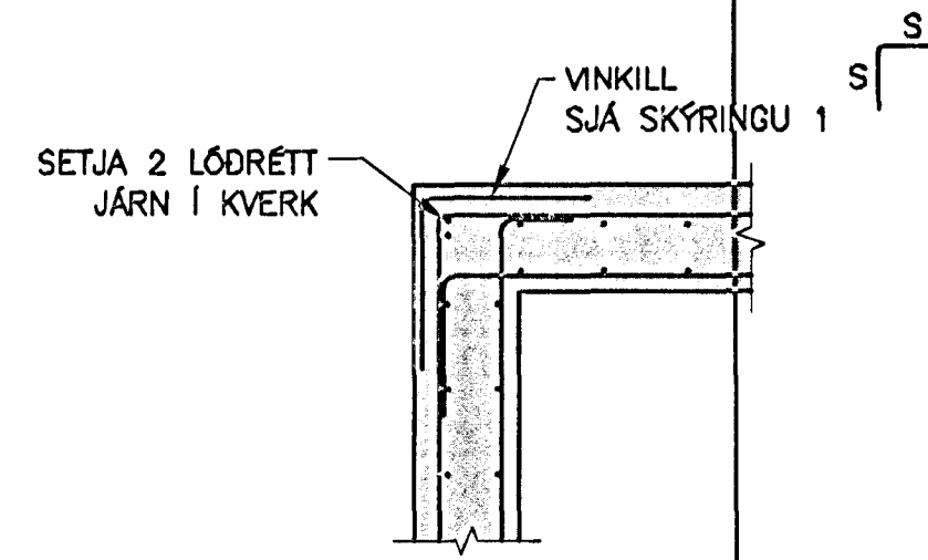
D01 DÆMIGERD JÁRNBENDING Í VEGG - LÁRÉTT SNID MKV. 1
