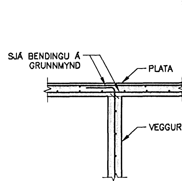
D01 DÆMIGERD JÁRNBENDING Í VEGG - LÁRÉTT SNID MKV. 1
