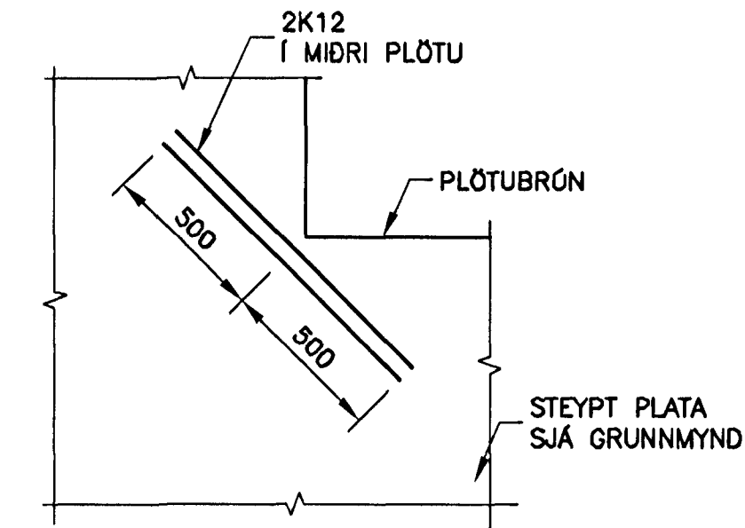
D06 JÁRNBENDING Í PLÖTUHÖRNI MKV. 1
