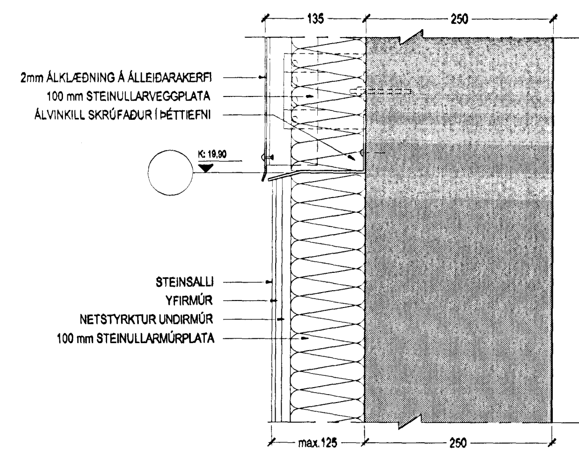
DEILI 9 - FRÁGANGUR VIÐ SKIL MILLI ÁL- OG MÚRKLÆÐNINGAR
