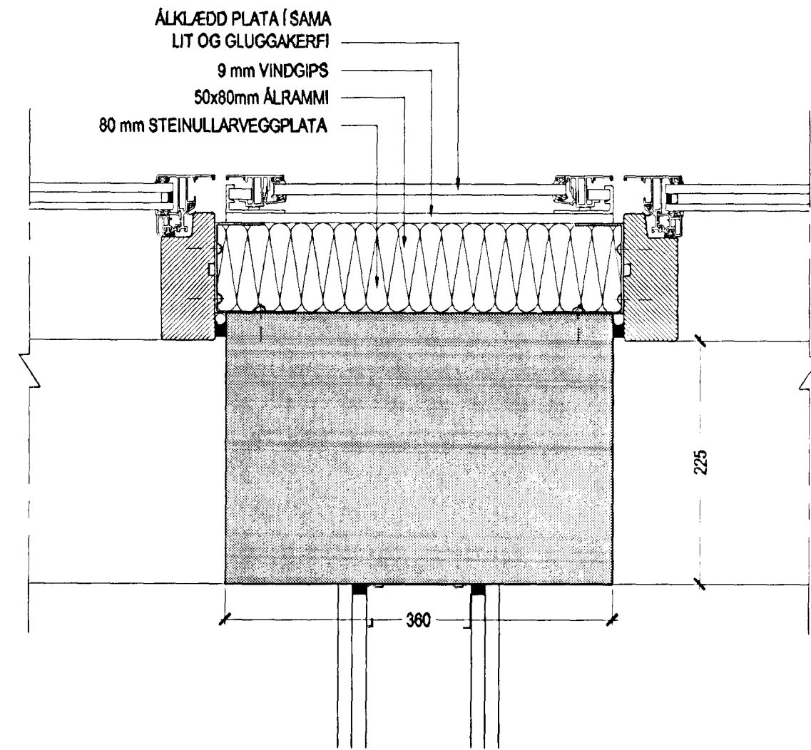
DEILI A - FRÁGANGUR ÞAR SEM GLUGGAKERFI GENGUR YFIR STEYPTA VEGGI
