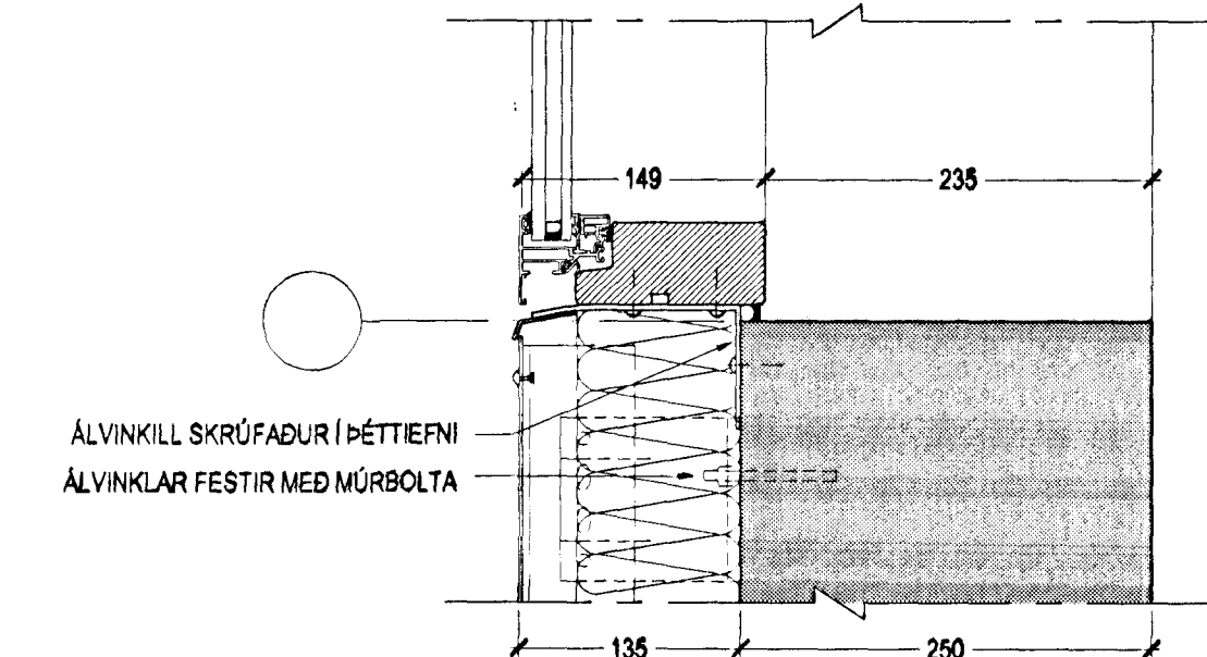
DEILI 3 - FRÁGANGUR VIÐ NEDRI BRÚN GLUGGA Á ÁLKLÆDDUM FLÖTUM
