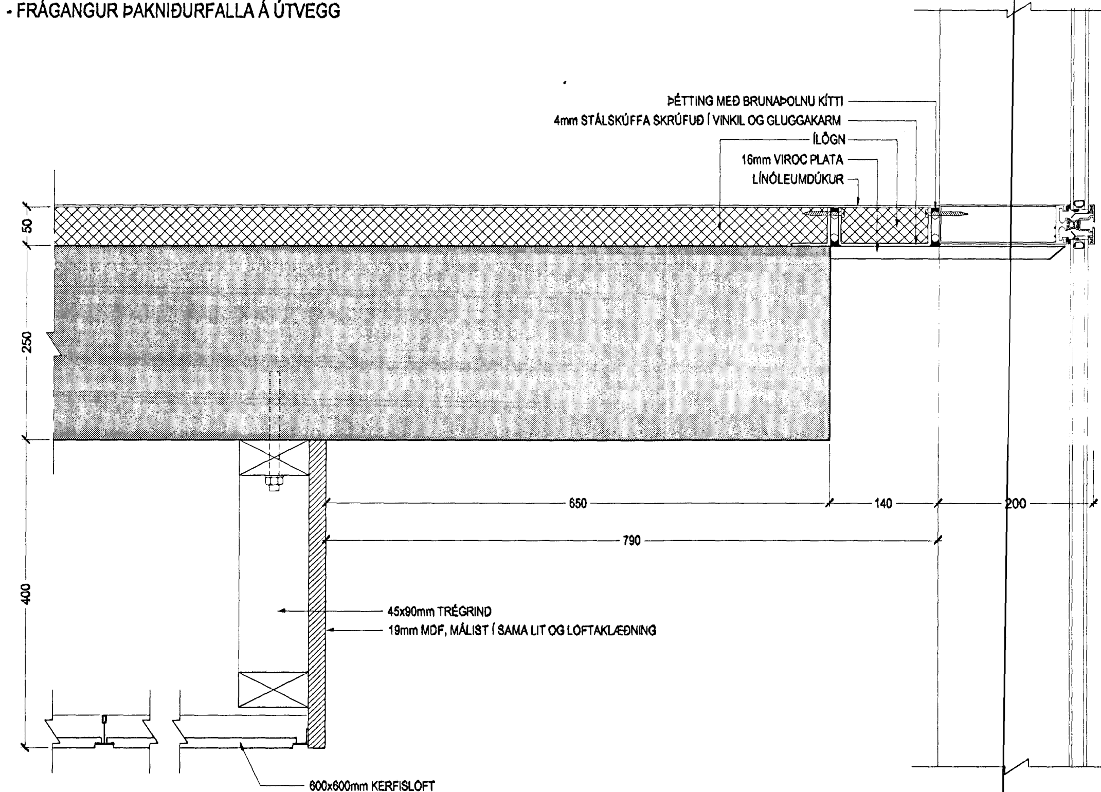
DEILI 10 - FRÁGANGUR VIÐ MILLIPLÖTU OG GLUGGAHLIÐ ANDDYRIS
