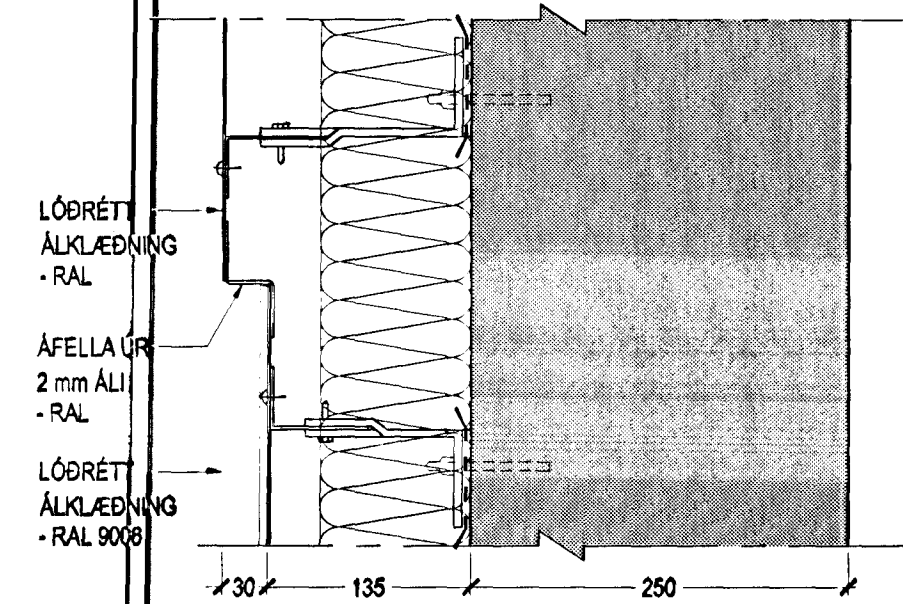
DEILI C - FRÁGANGUR VIÐ ÚTKRÖKUN ÁLKLÆÐNINGAR VIÐ FYRIRLESTRARSAL
