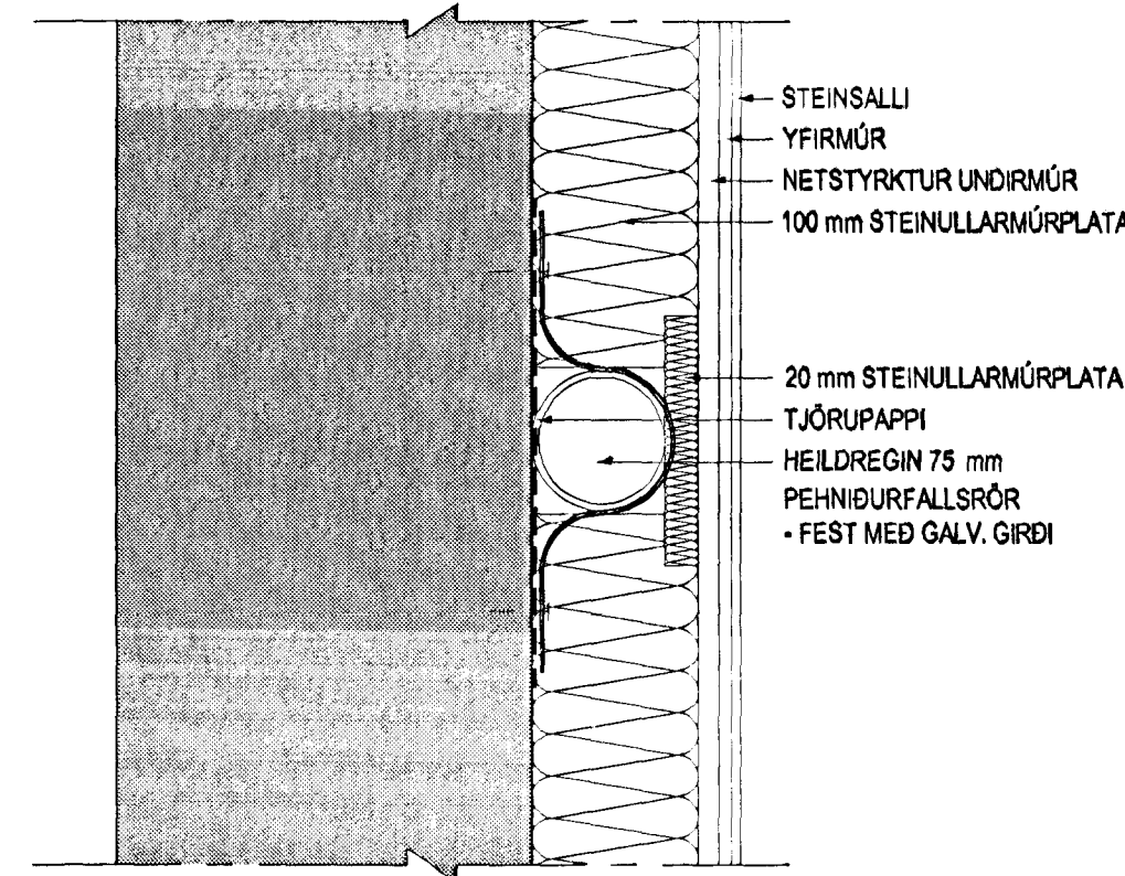
DEILI F - FRÁGANGUR ÞAKNIÐURFALLA Á ÚTVEGG
