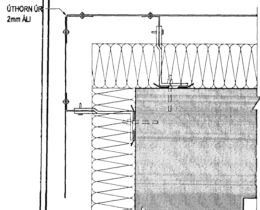
DEILI B - ALMENNUR FRÁGANGUR VIÐ ÚTHORN LÓÐRÉTTRAR KLÆÐNINGAR
