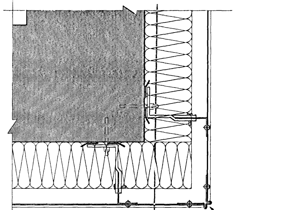
DEILI E - ALMENNUR FRÁGANGUR VIÐ ÚTHORN
