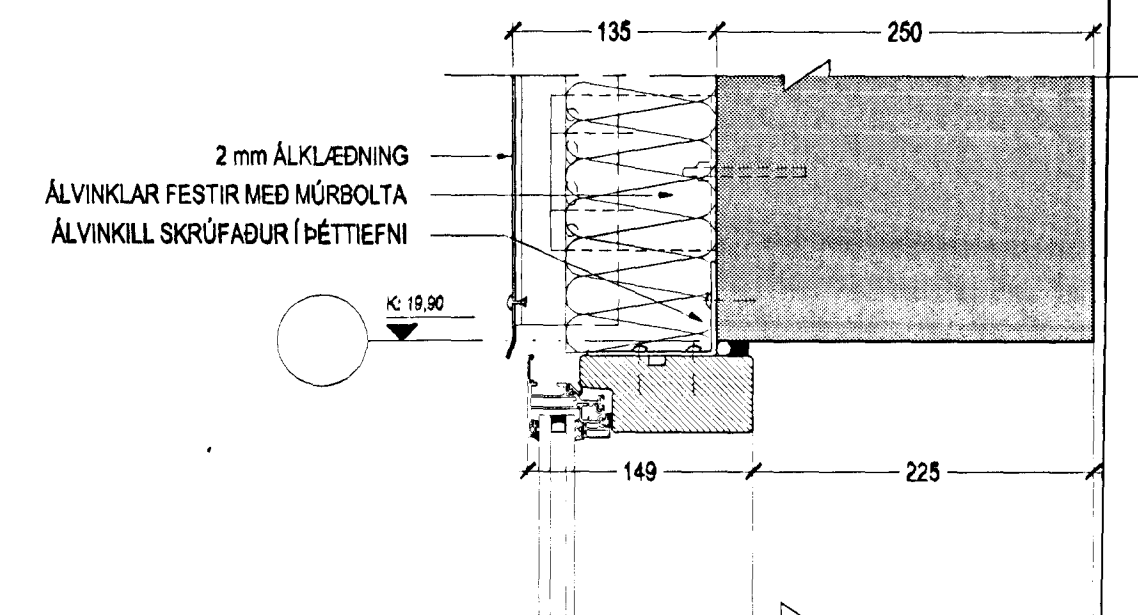
DEILI 2 - FRÁGANGUR VIÐ EFRI BRÚN GLUGGA Á MÚRHÚÐUÐUM FLÖTUM
