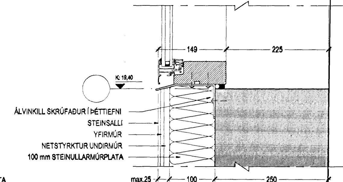
DEILI 1 - FRÁGANGUR VIÐ BOTN- OG HLIÐARSTYKKI GLUGGA Á MÚRHÚÐUÐUM FLÖTUM
