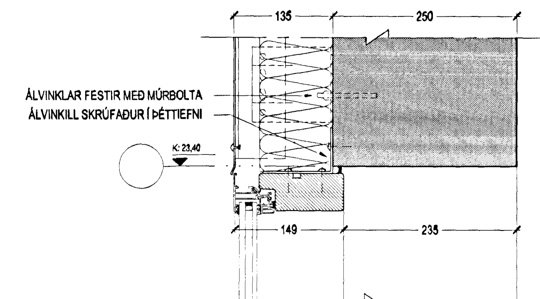
DEILI 4 - FRÁGANGUR VIÐ EFRI BRÚN GLUGGA Á ÁLKLÆDDUM FLÖTUM
