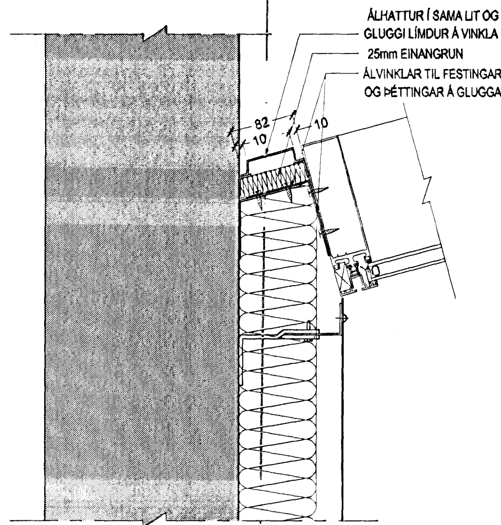
DEILI D - FRÁGANGUR VIÐ GLUGGAVEGG
