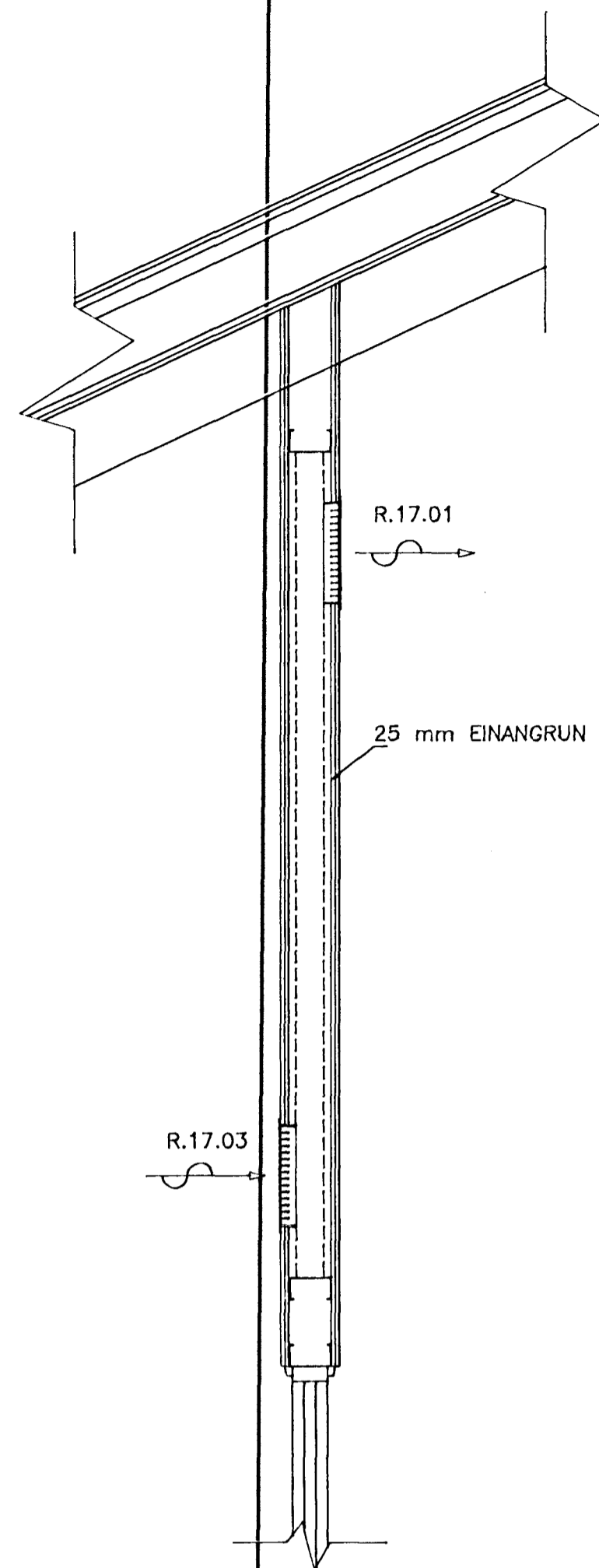
7 0413 SNID 1:20
