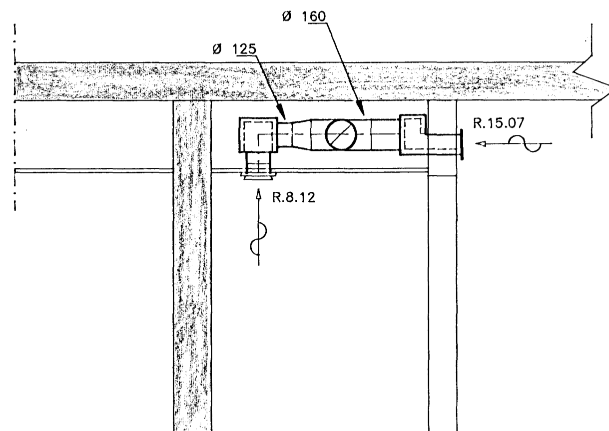
11 0413 SNID 1:20
