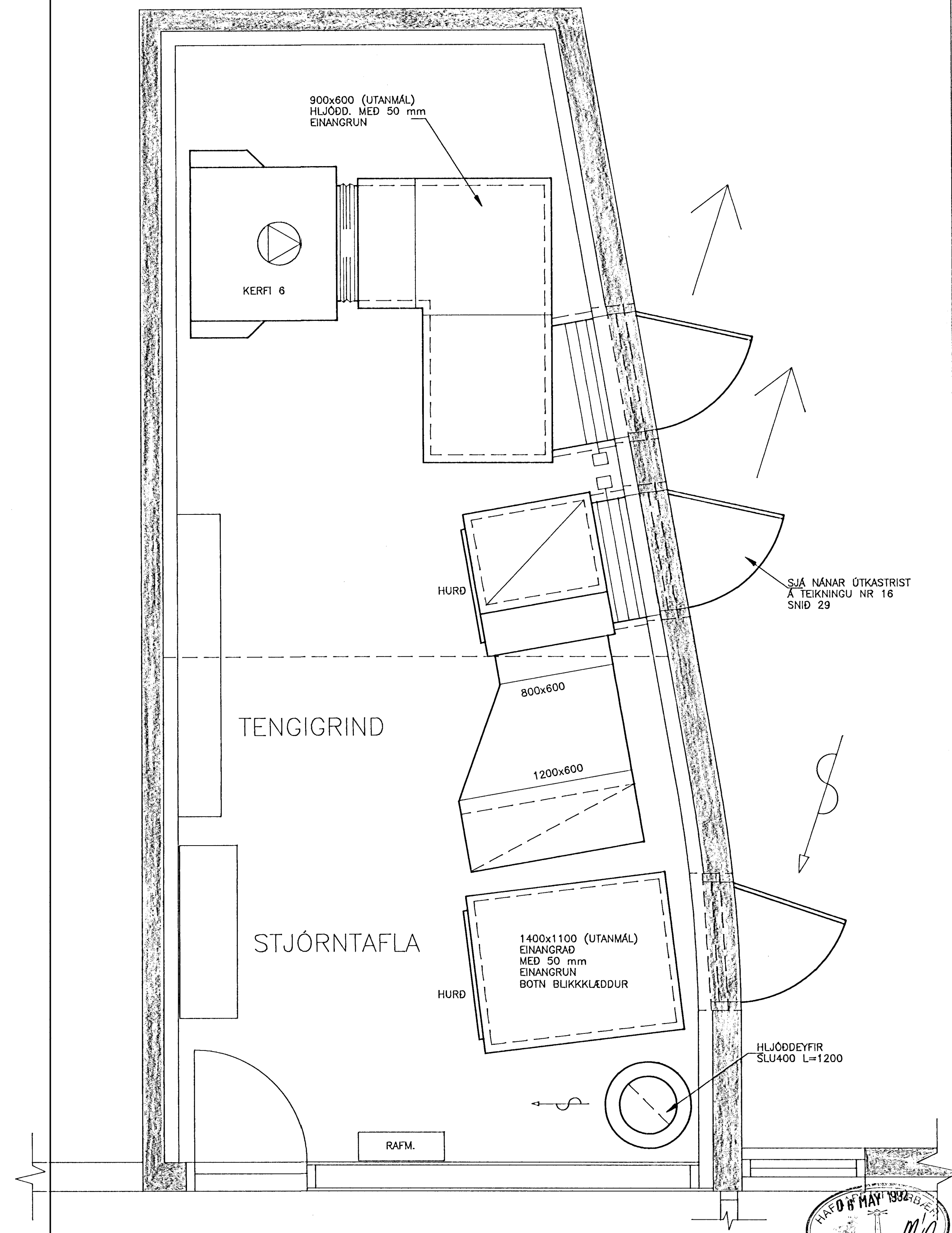
GRUNNMYND 2 1:20 (MIDHLUTI)
