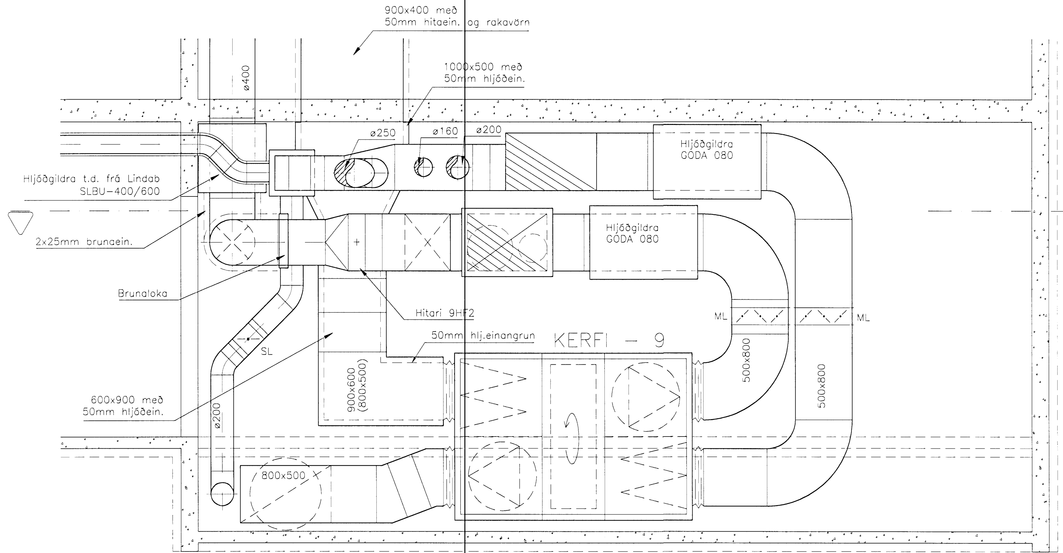
1 Snið 02/06 03 Mkv. 1: 20
