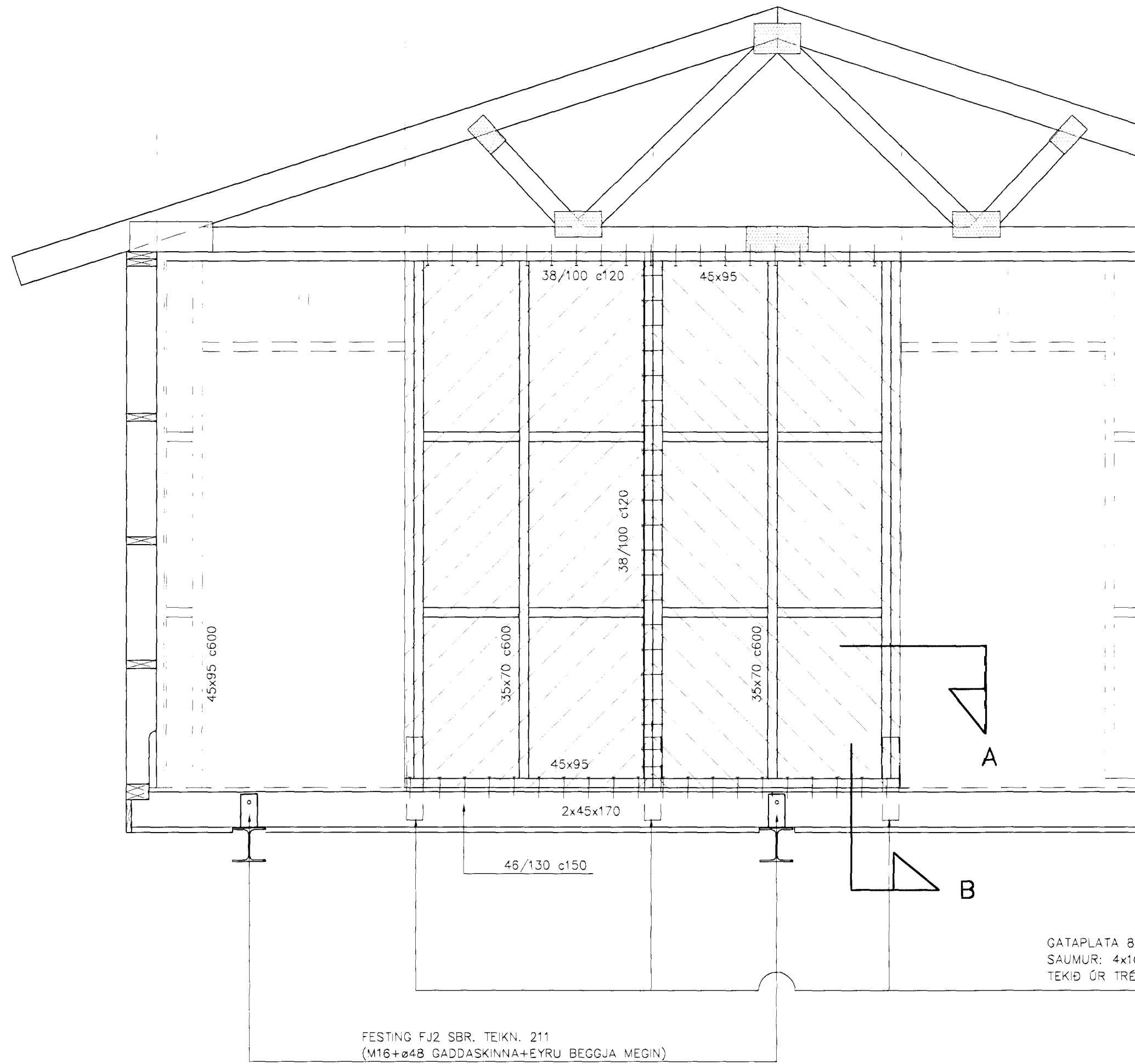
STÍFINGARINNVEGGUR Mkv. 1:20
