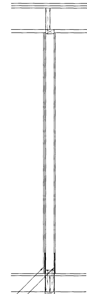
SNÍÐ B Mkv. 1:10
