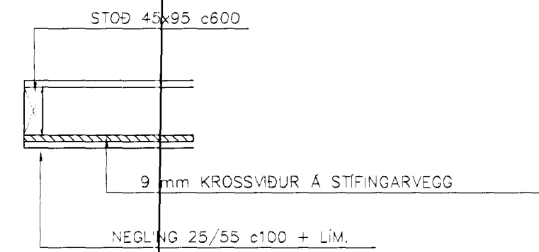
SNÍÐ A (TENGING VIÐ LÍMTRÉSSÓLU) Mkv. 1:10
