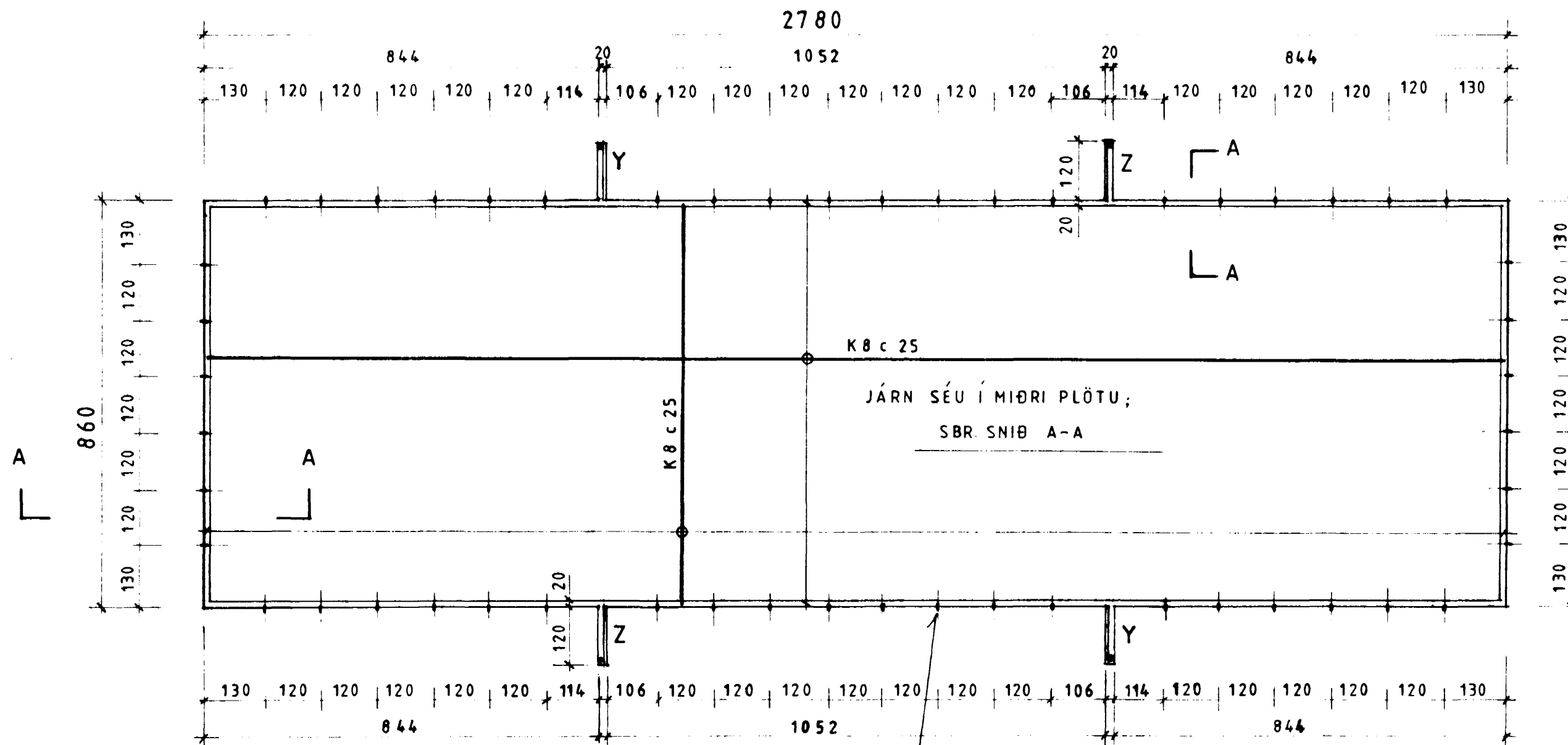
GRUNNMYND M=1:100
