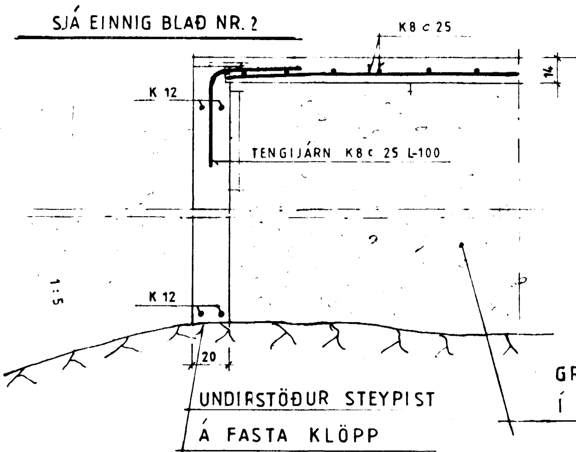
SNÍÐ A-A M=1:20; UNDIRSTÖÐUR
