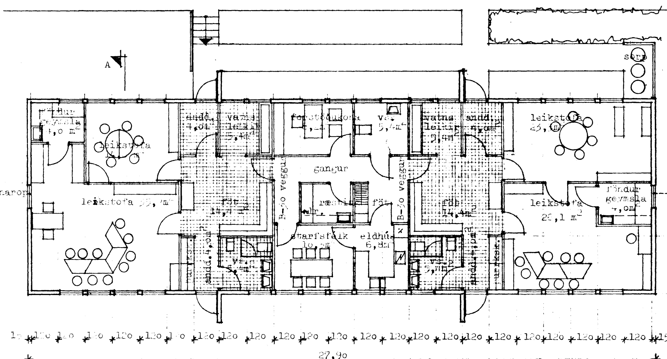
grunnmynd
