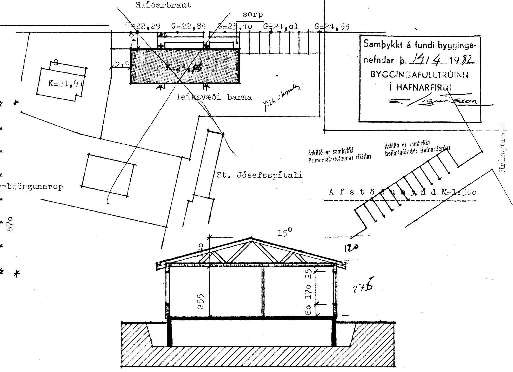
skurður A-A
