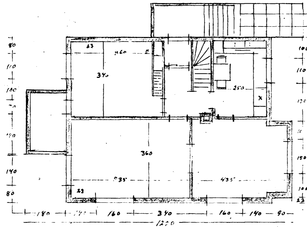
1. hæð
