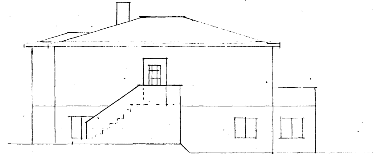
Norðurlíð
