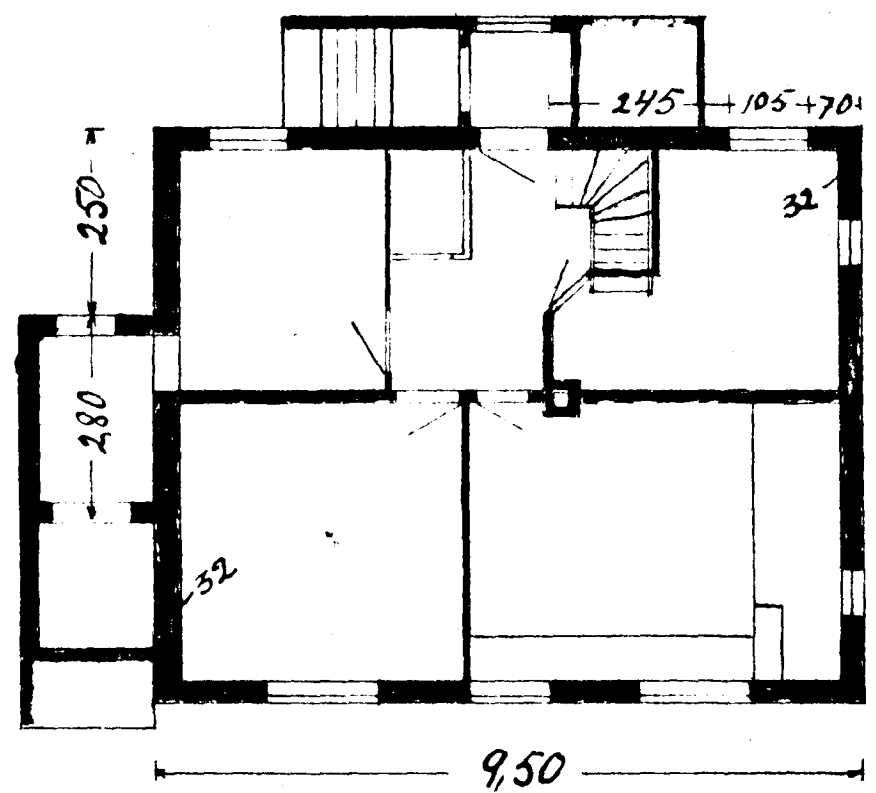
KJALLARI.
