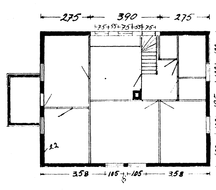
ÞAK HÆÐ.
