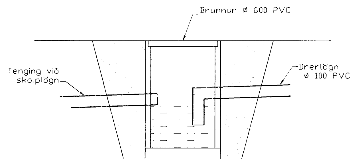
Vatnslásabrunnur, 1:20
