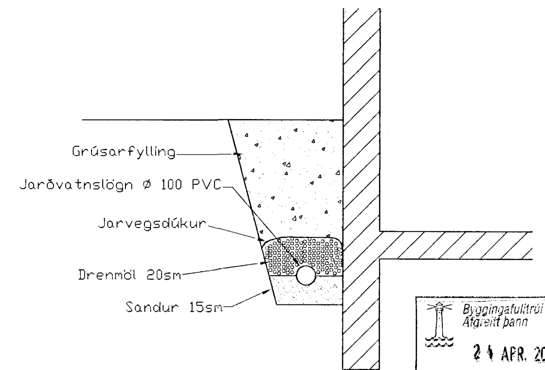
Drenlög, Snið 1:20
