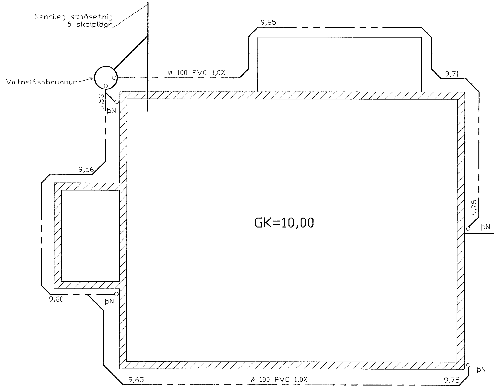
Drenlög, Grunnmynd 1:50
