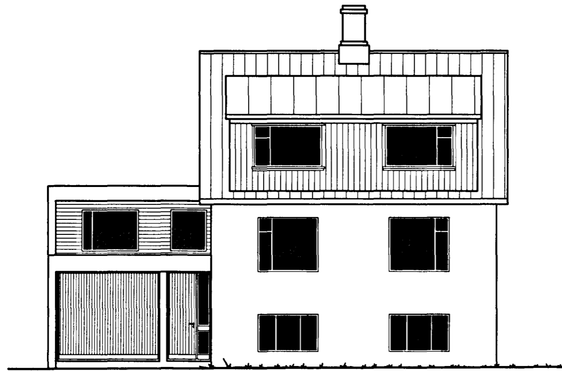
ÚTLIT VESTUR 1:100
