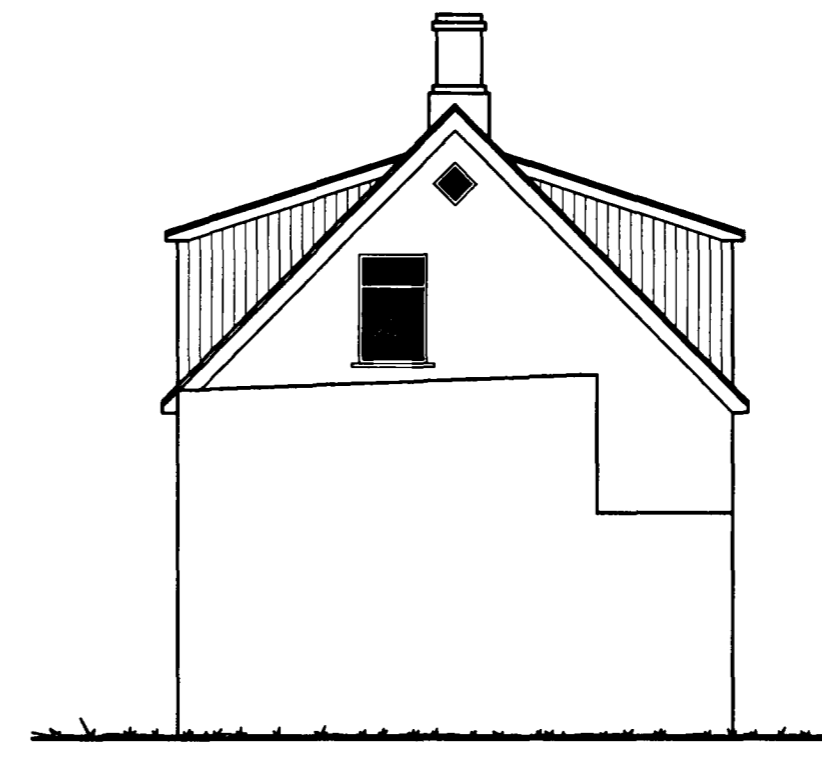
ÚTLIT NORÐUR 1:100
