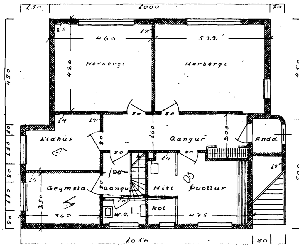
1. hæð
