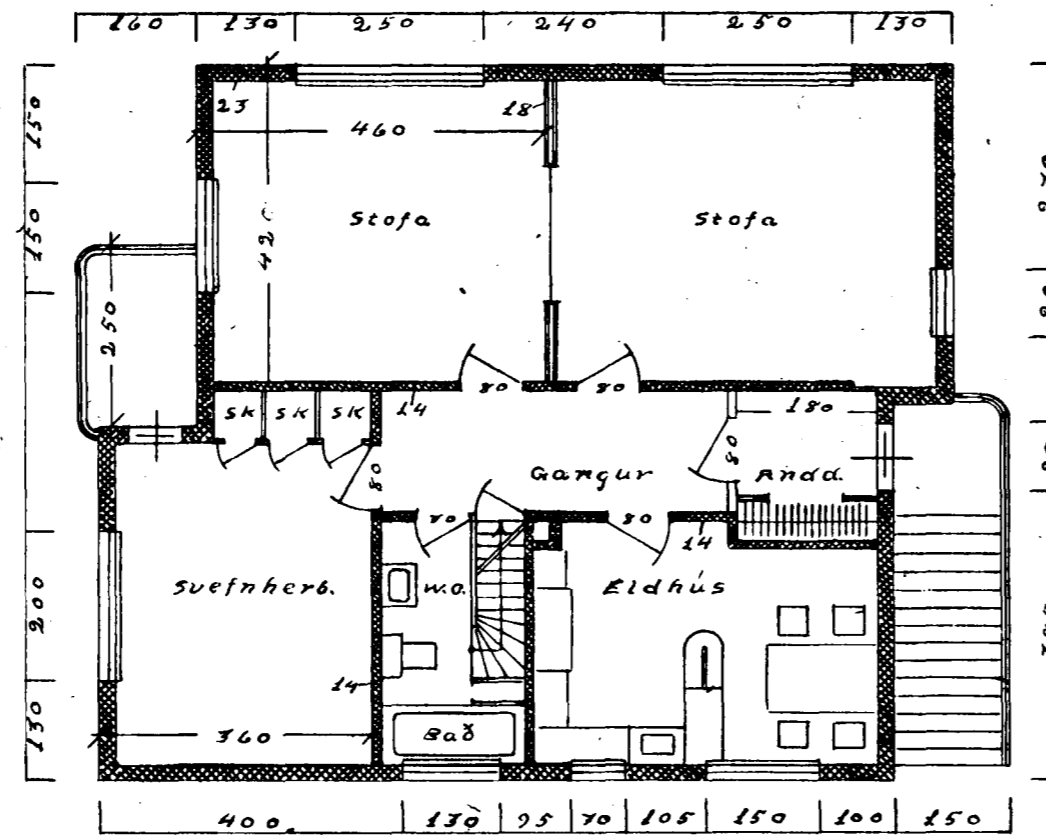
2. hæð
