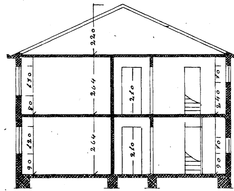
Skurður
