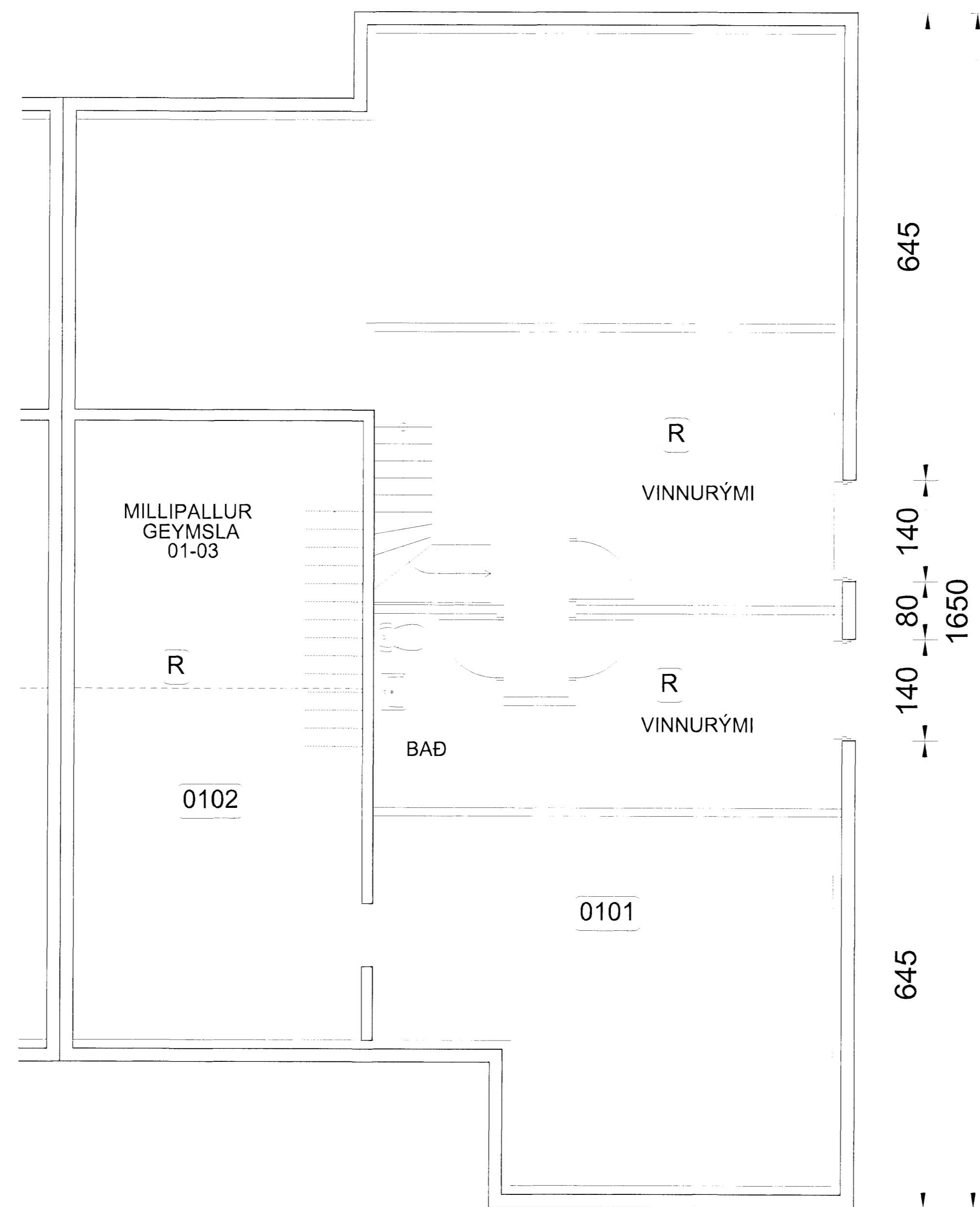
GRUNNMYND HÚS 31, 2. HÆÐ 1:50
