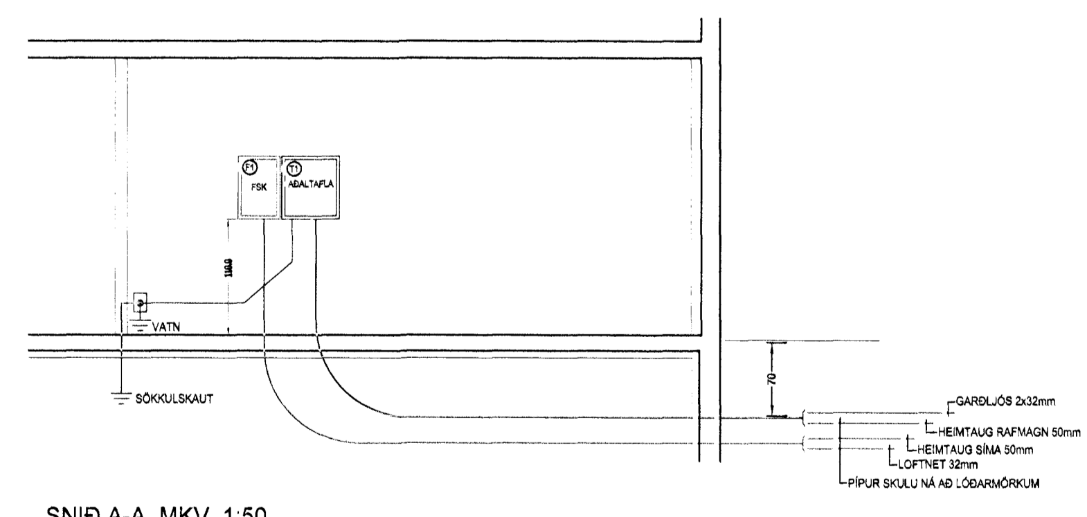
SNIÐ A-A MKV. 1:50
