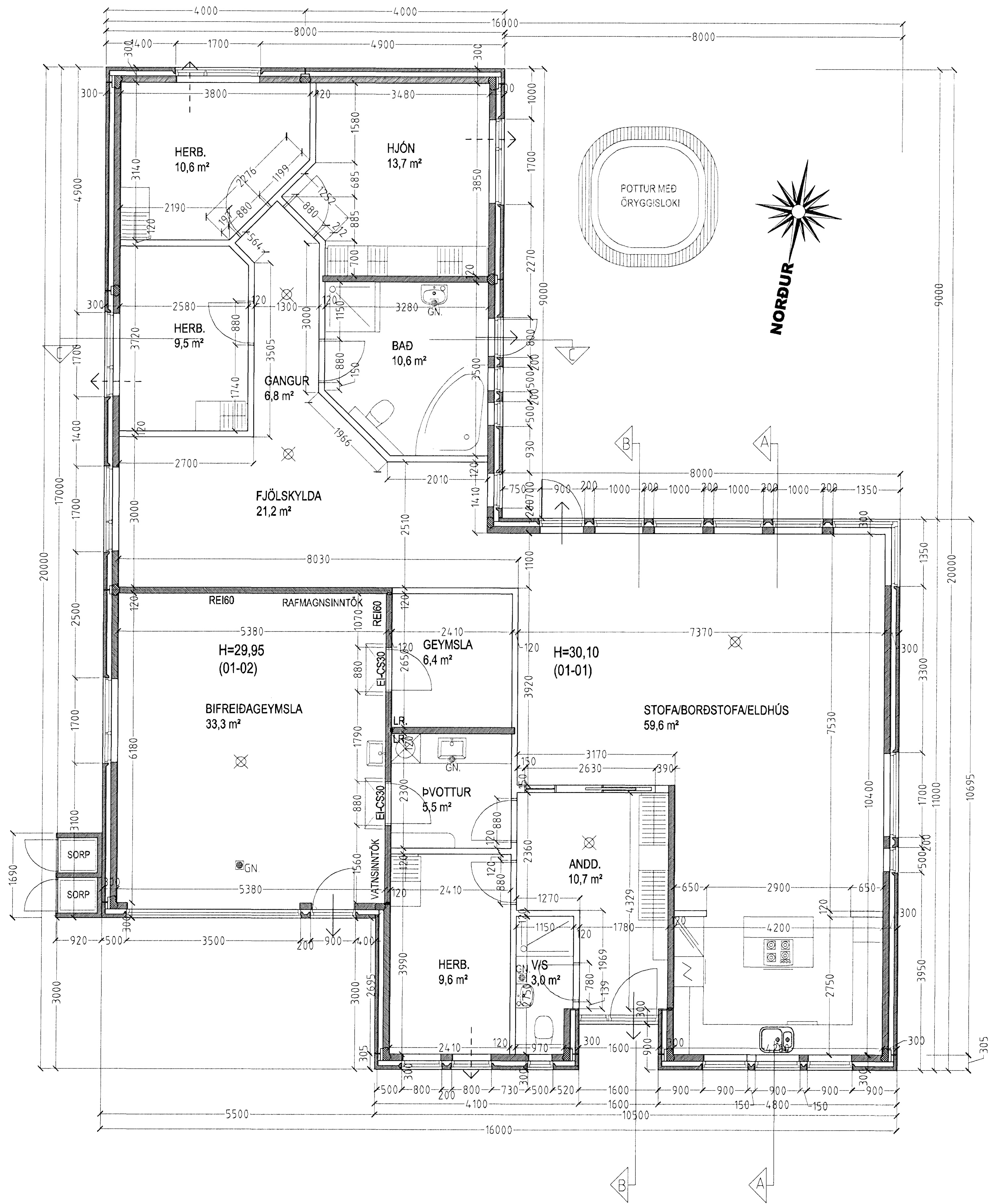
GRUNNMYND 1. HÆÐ MKV. 1:50.
