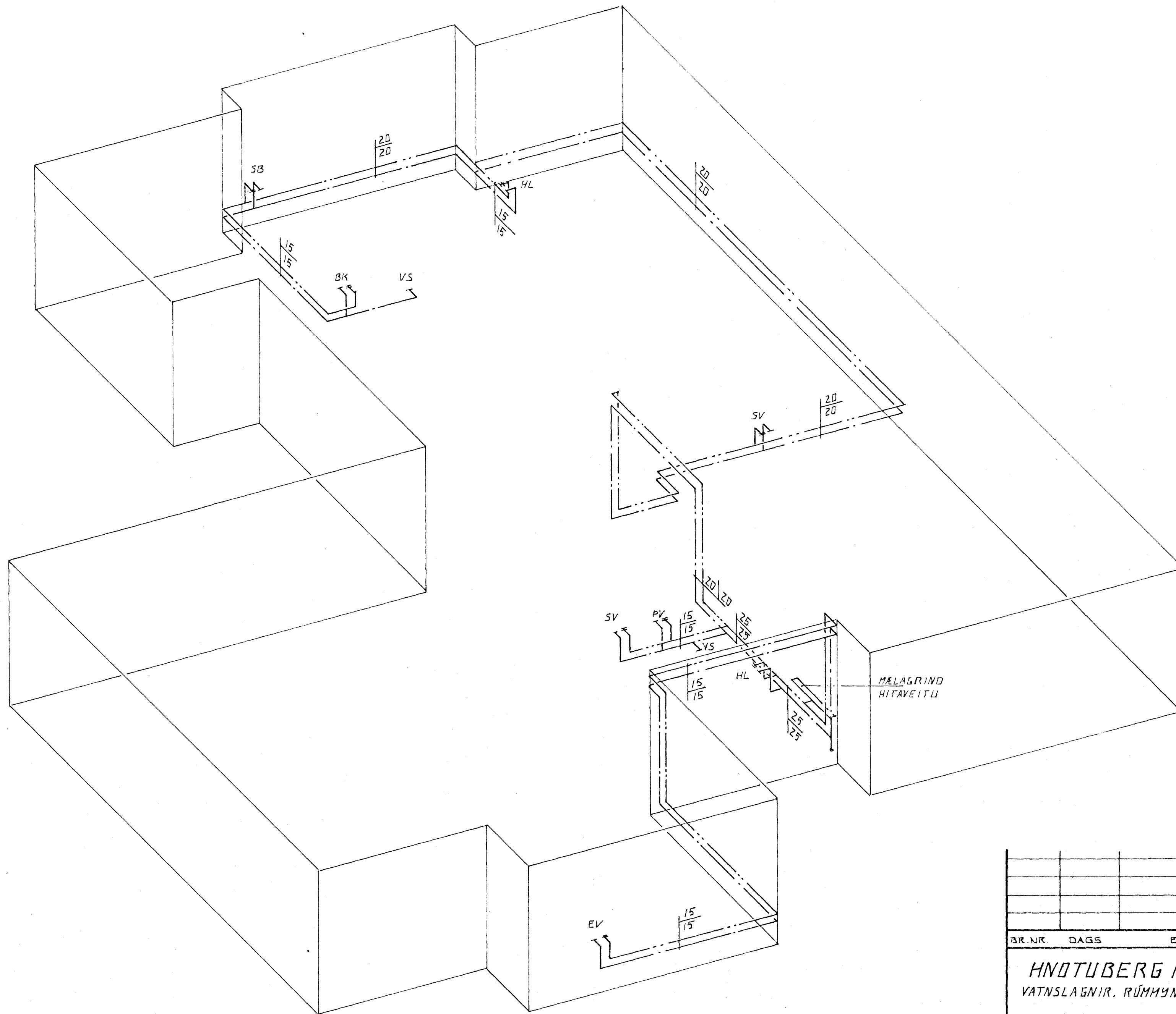
RÚMMYND 1:50
