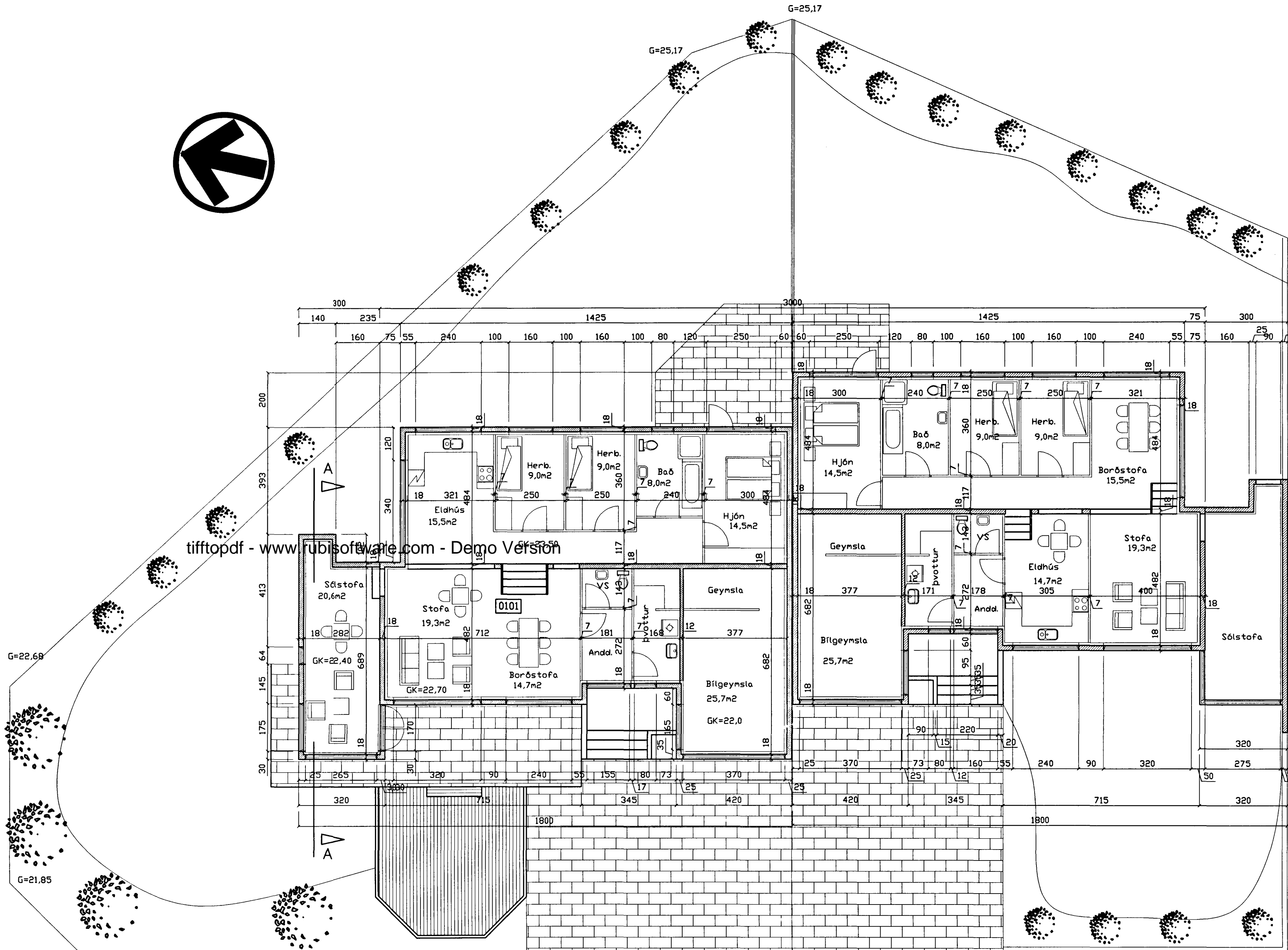
Grunnmynd, 1:100
