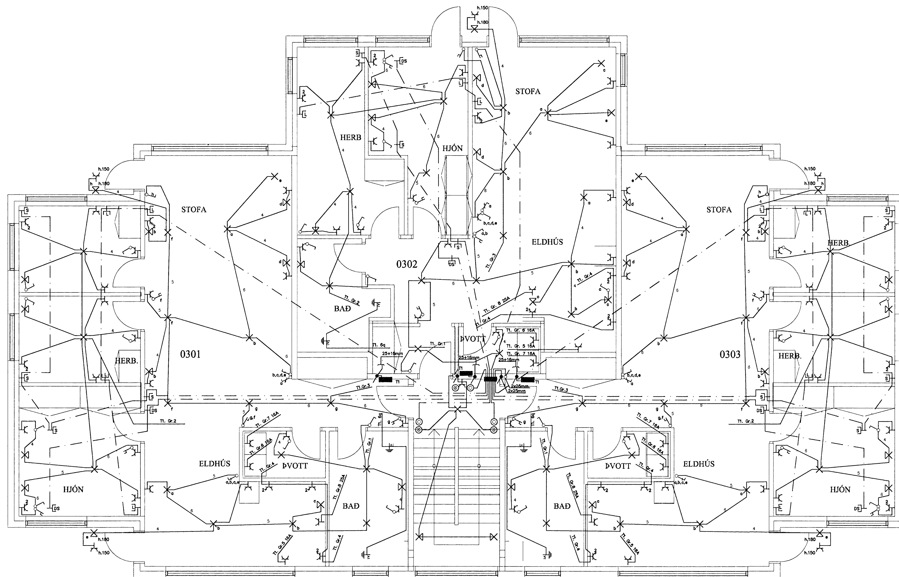
Grunnmynd 3 hæðar
