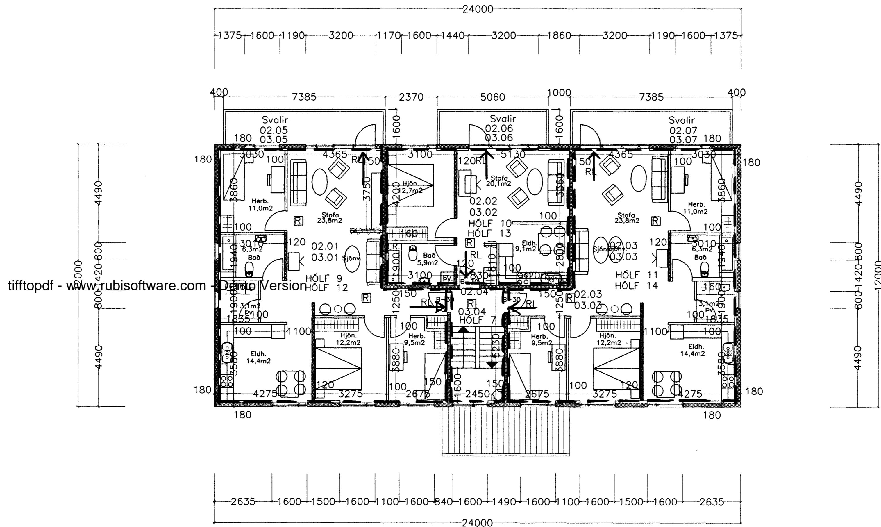
Grunnmynd 2-3 Hæðar
