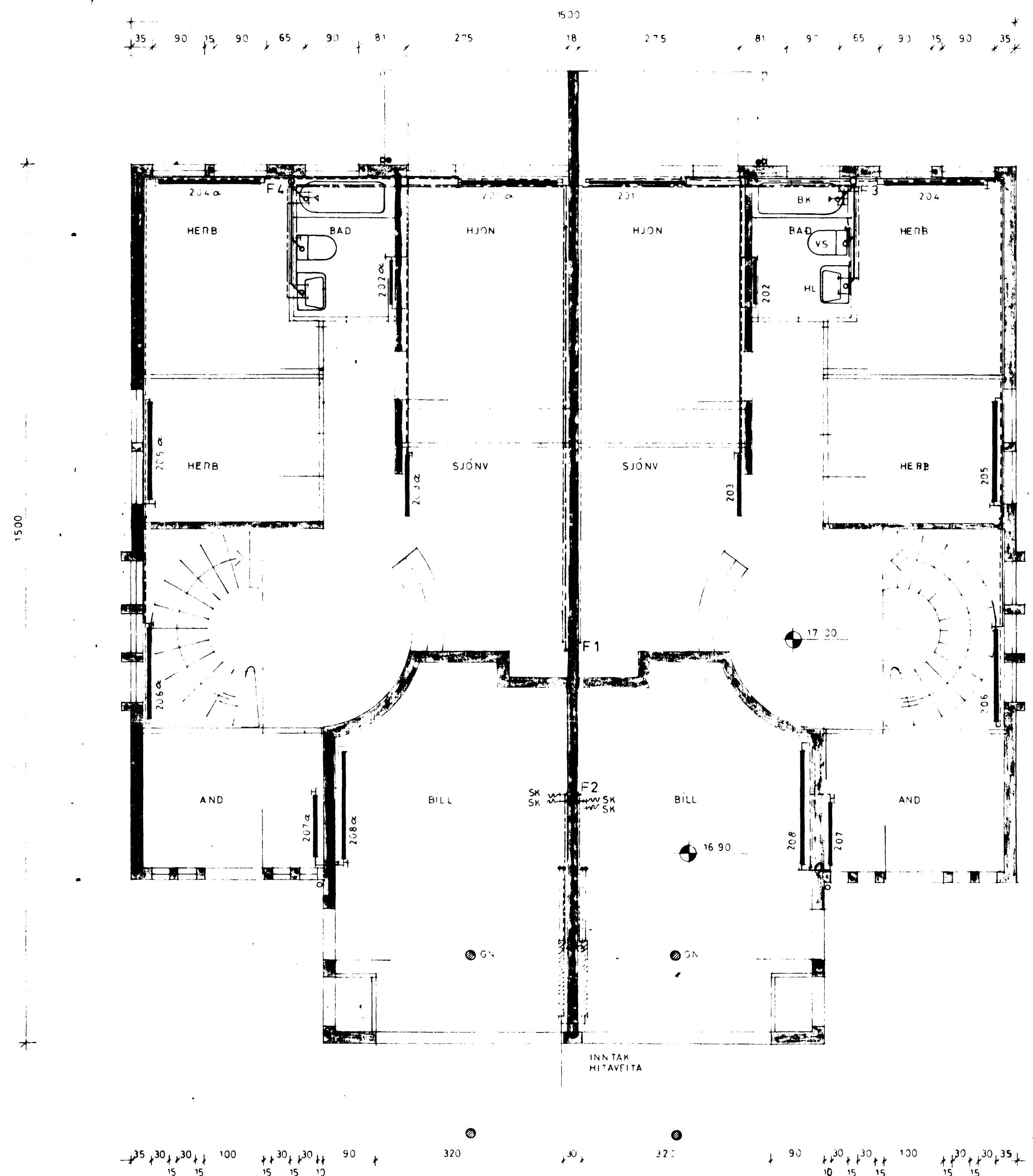
GRUNNMYND 1 HÆÐ
