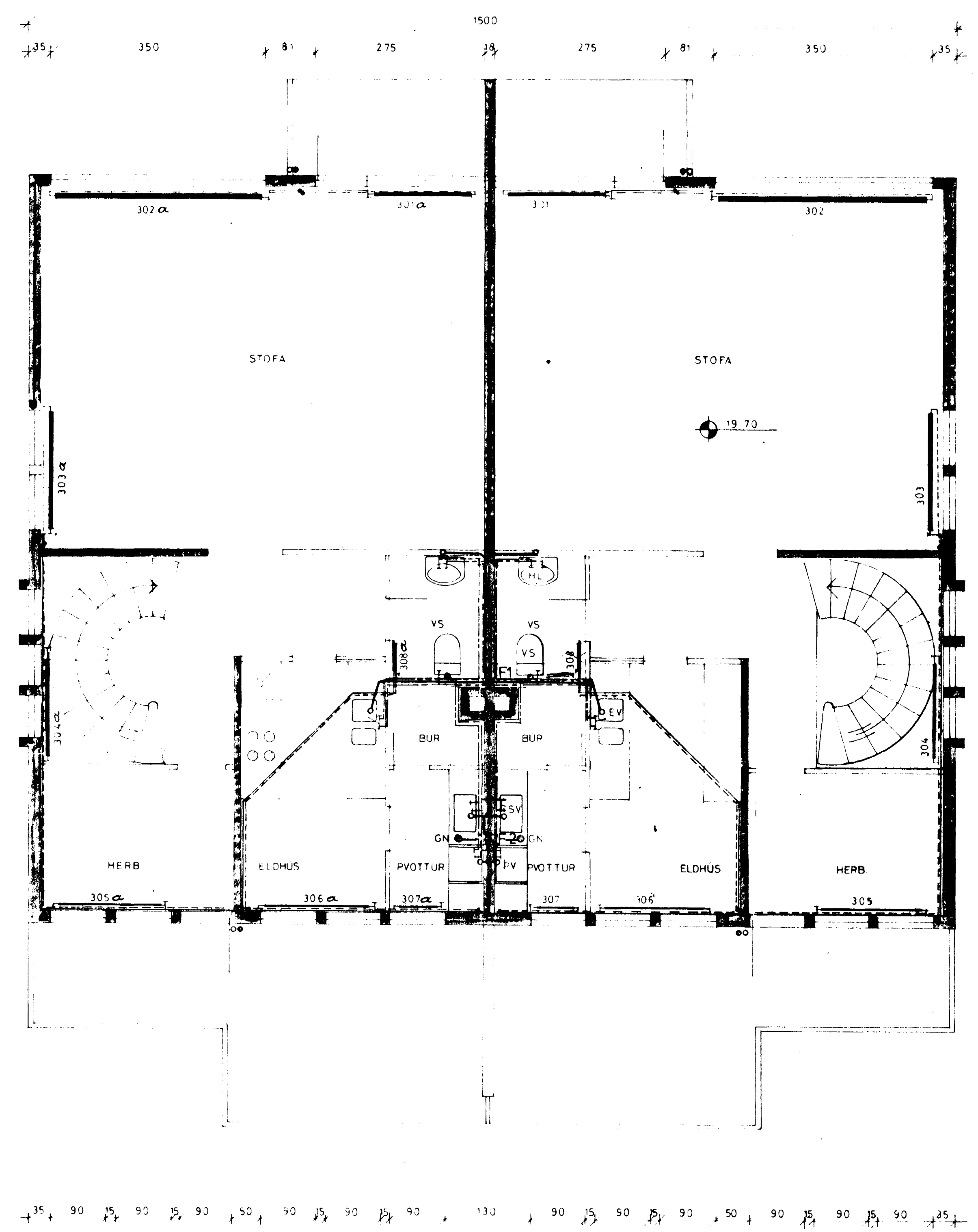
GRUNNMYND 2 HÆÐ
