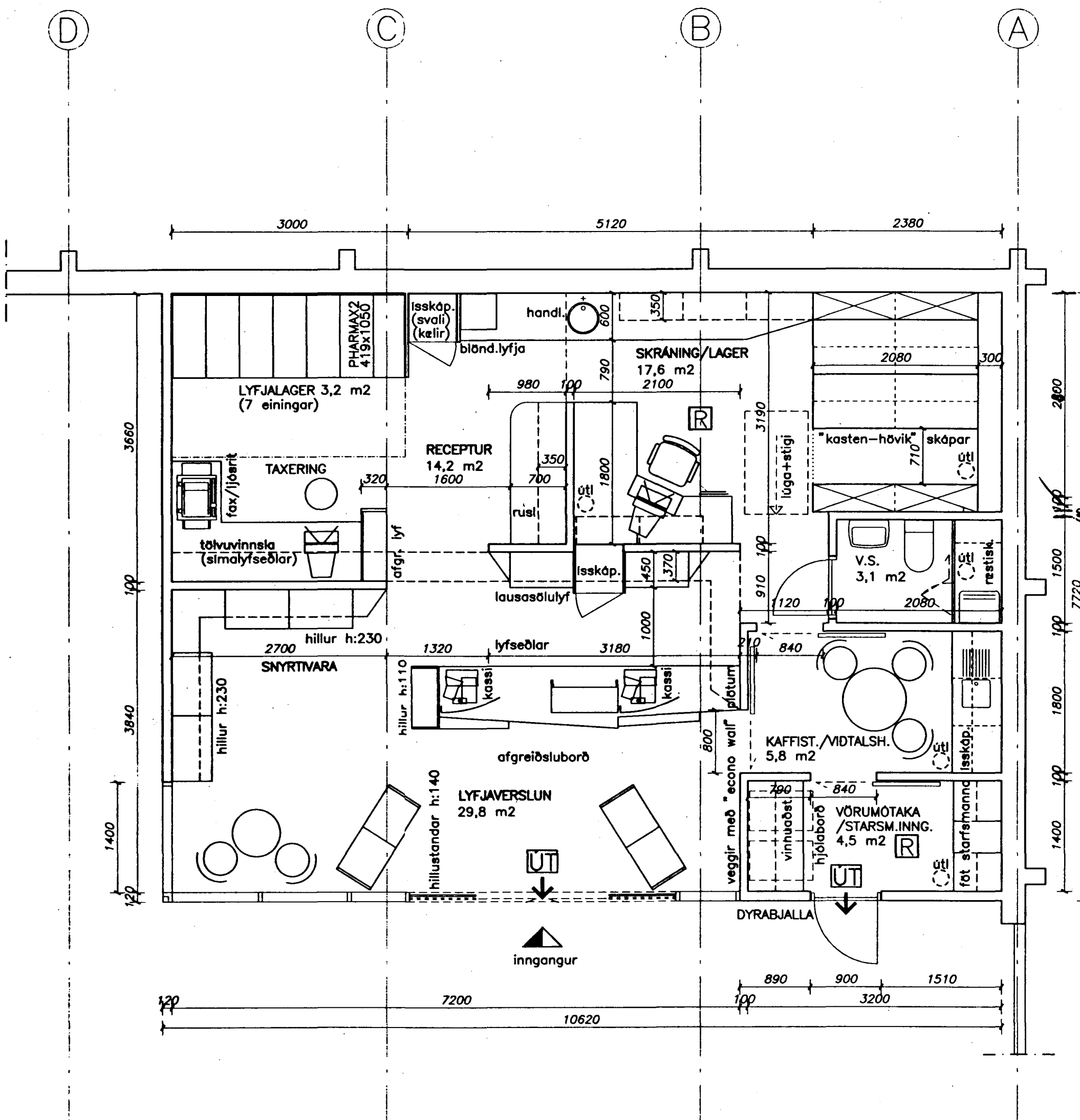
JARDHÆÐ 1:50
