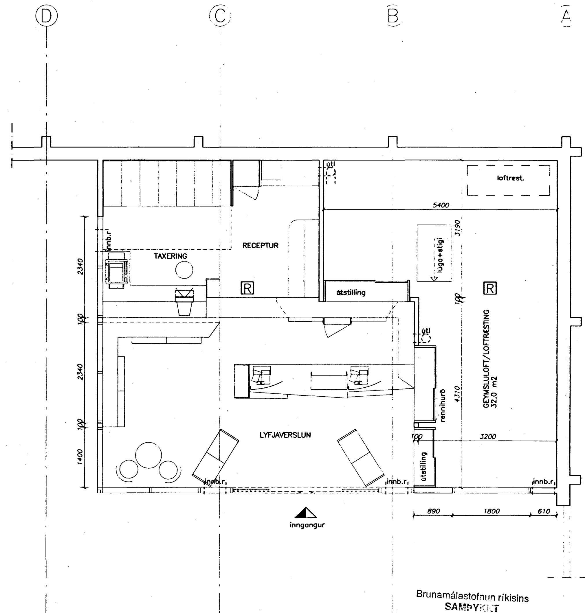
GEYMSLULOFT/ÚTSTILLING 1:50
