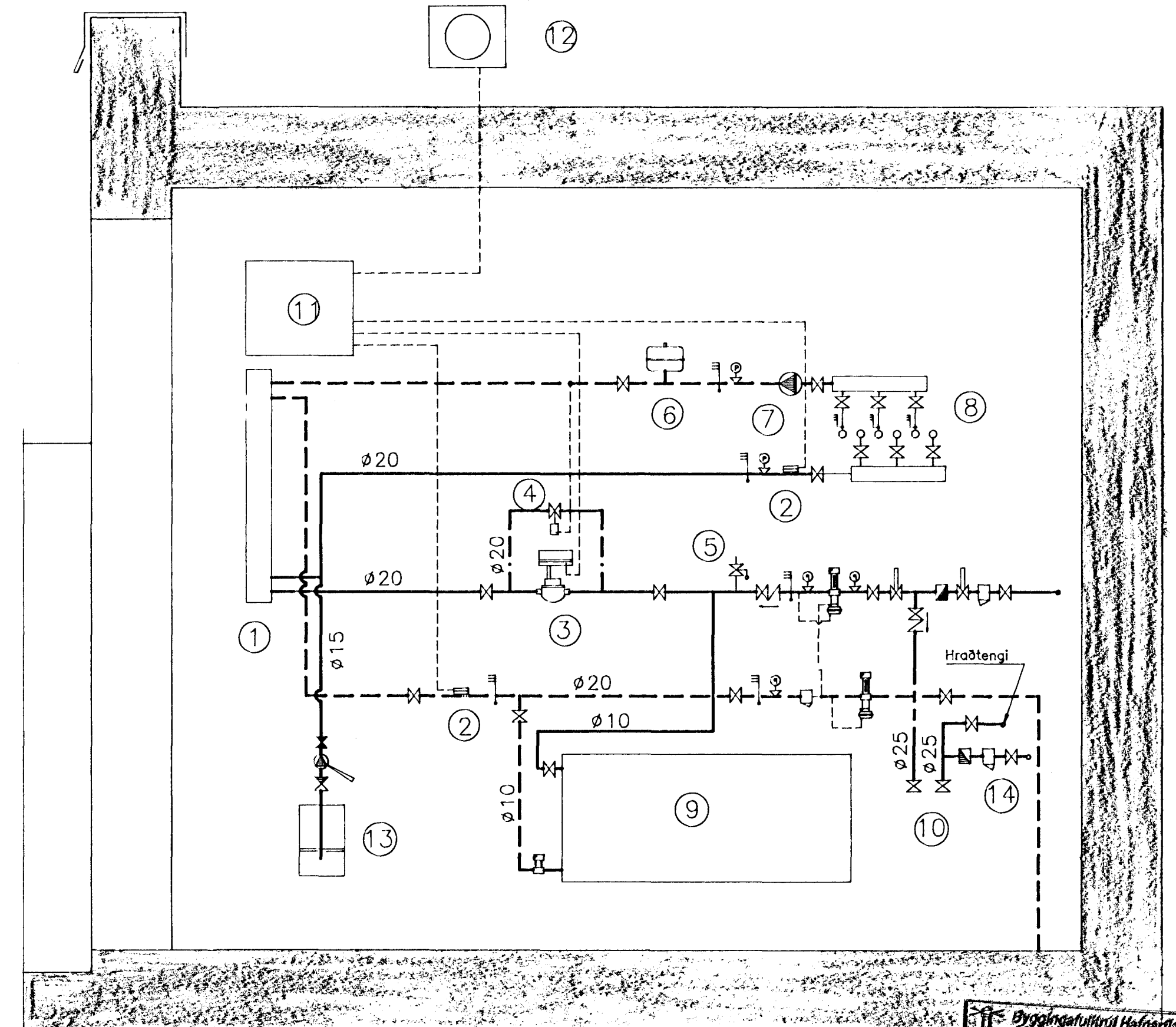
TENGIGRIND, STÝRINGAR, KERFISMYND 1:10
