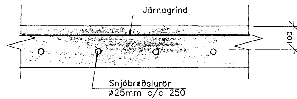
SNID I SNJÖBRÆDSLU 1:10
