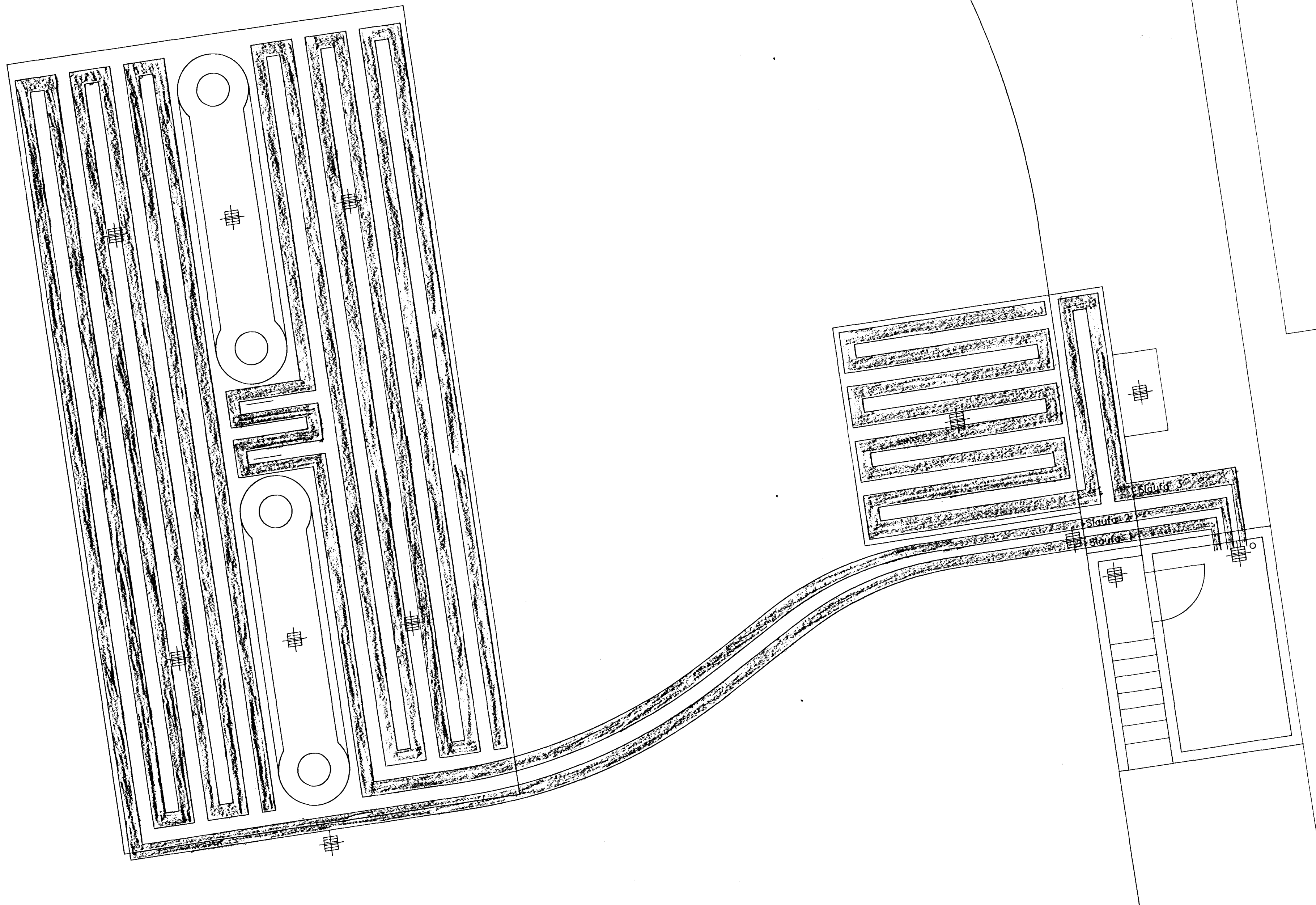
GRUNNMYND 1:50
