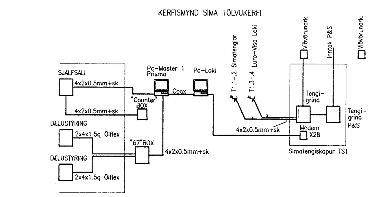
SMÁSPENNUKERFI KERFISMYND
