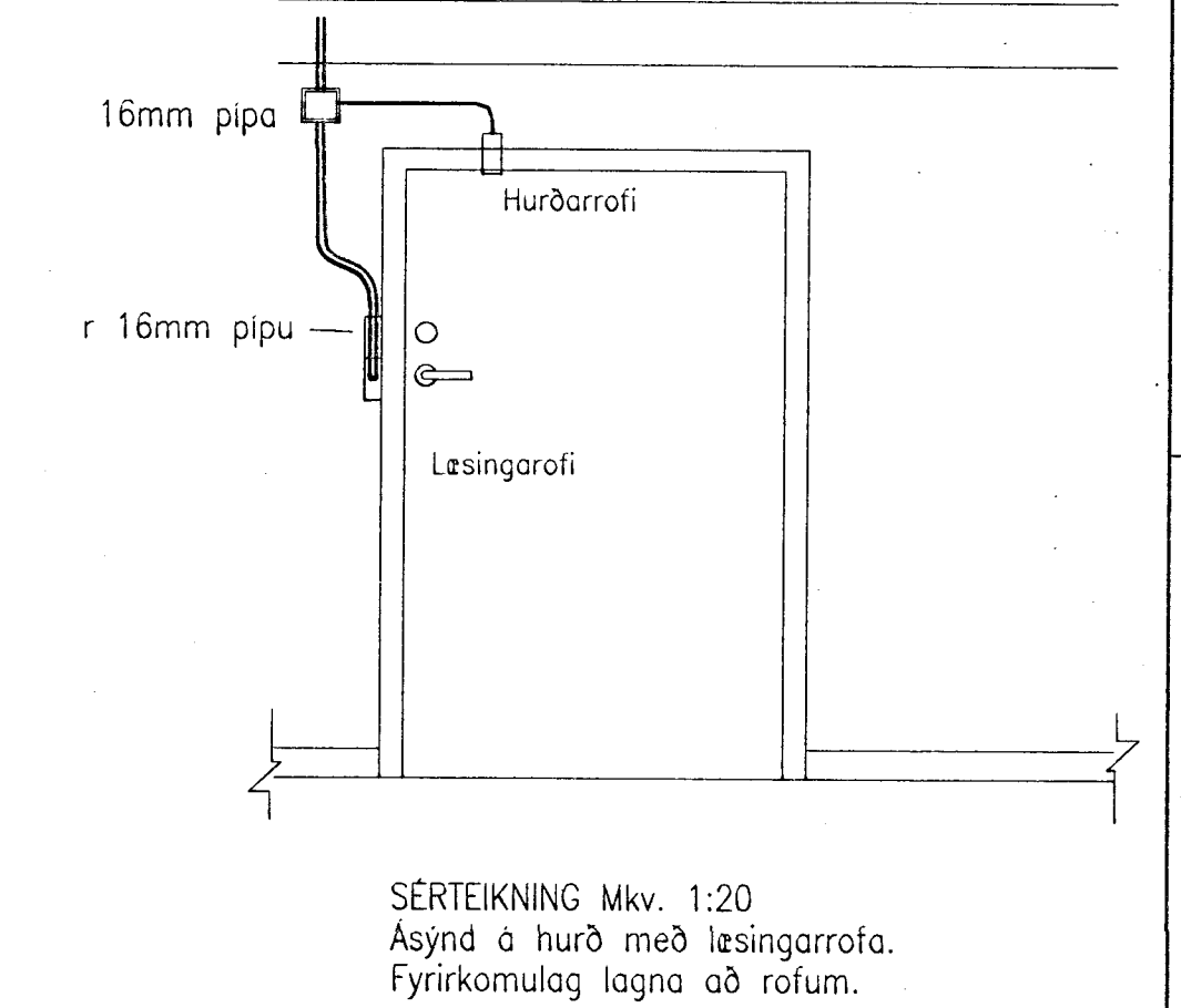
SERTEIKNING Mkv. 1:20
