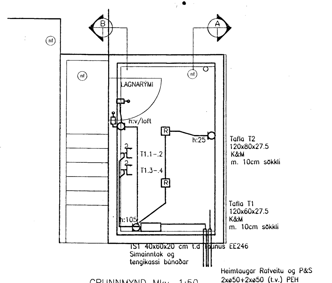
SMÁSPENNUKERFI
