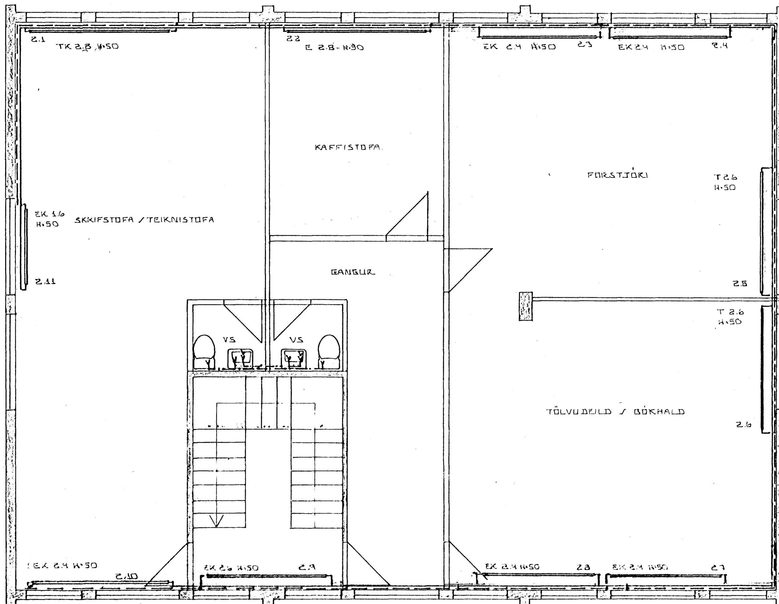
GRUNNMYND 2. HÆÐAR 1:50
