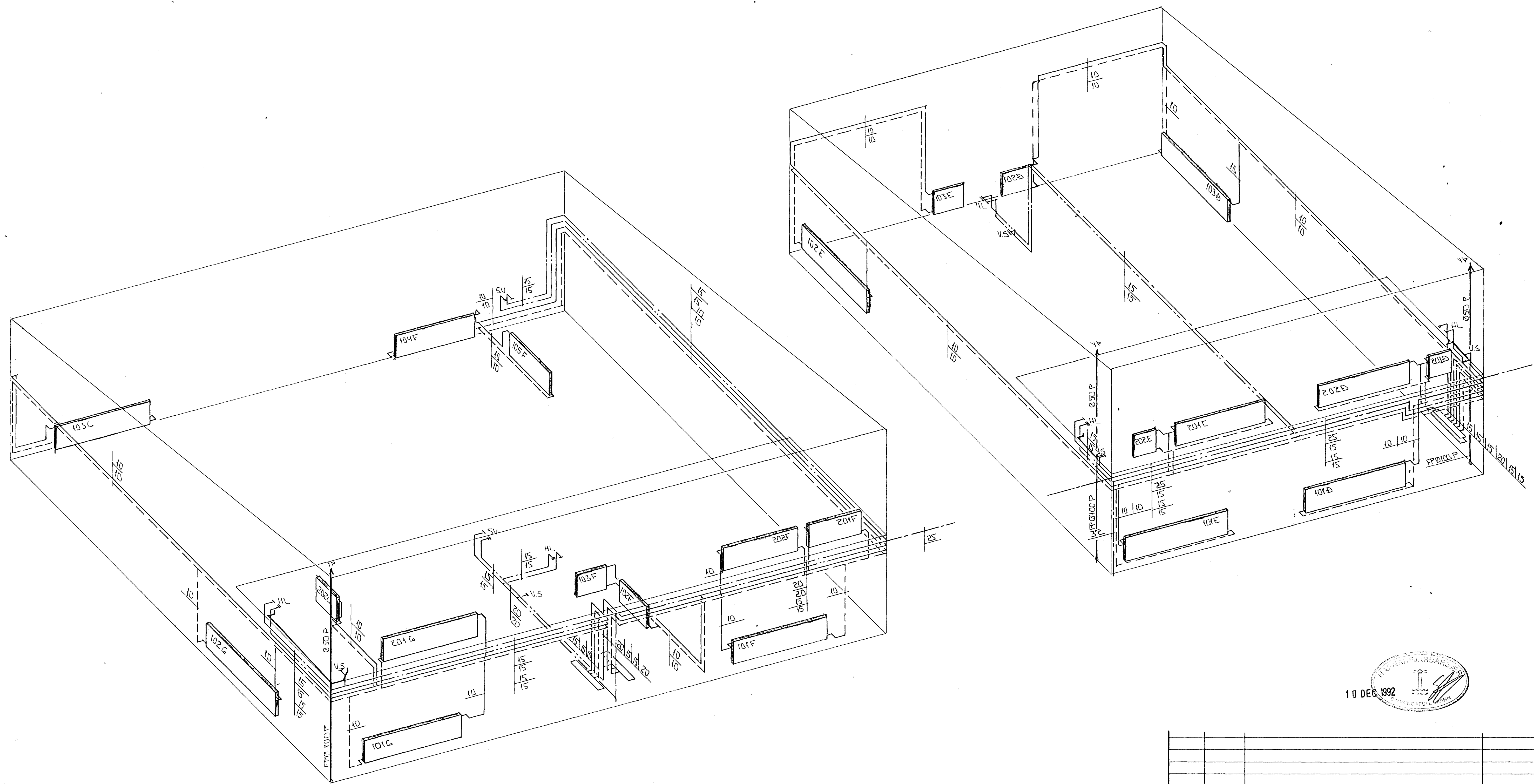
RÚMMYND 1:50
