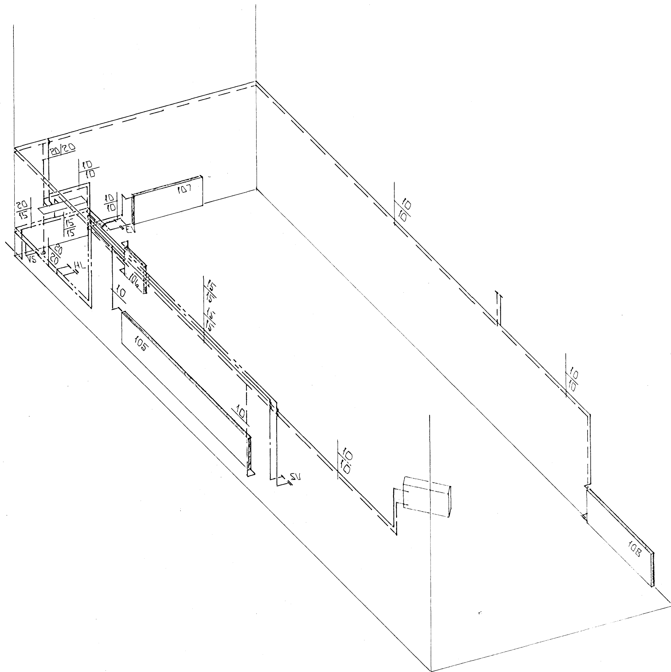
RÚMMYND BIL B x 1:50
