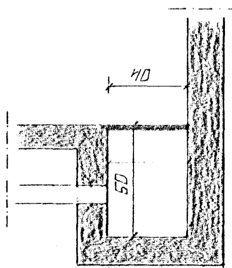
DÆLUÞRÚNNUR Í GRÝFJU. 1:20
