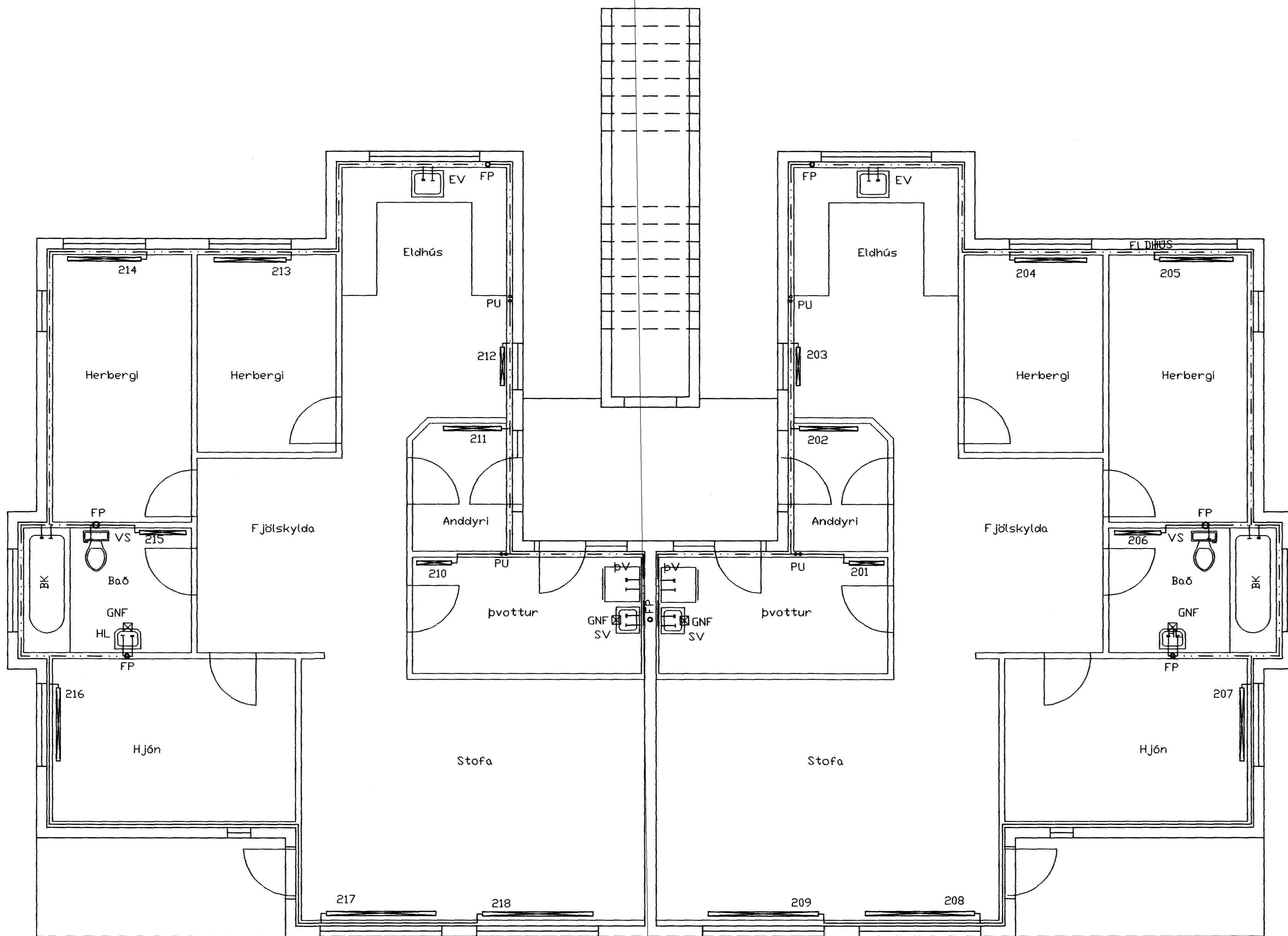
LAGNIR 2. HÆÐ, GRUNNMYND 1:50
