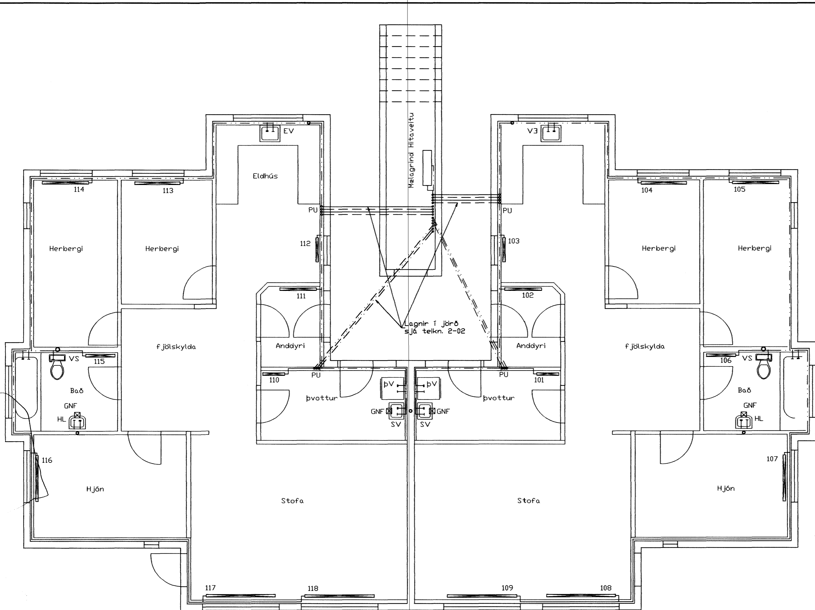
LAGNIR 1. HÆÐ, GRUNNMYND 1:50
