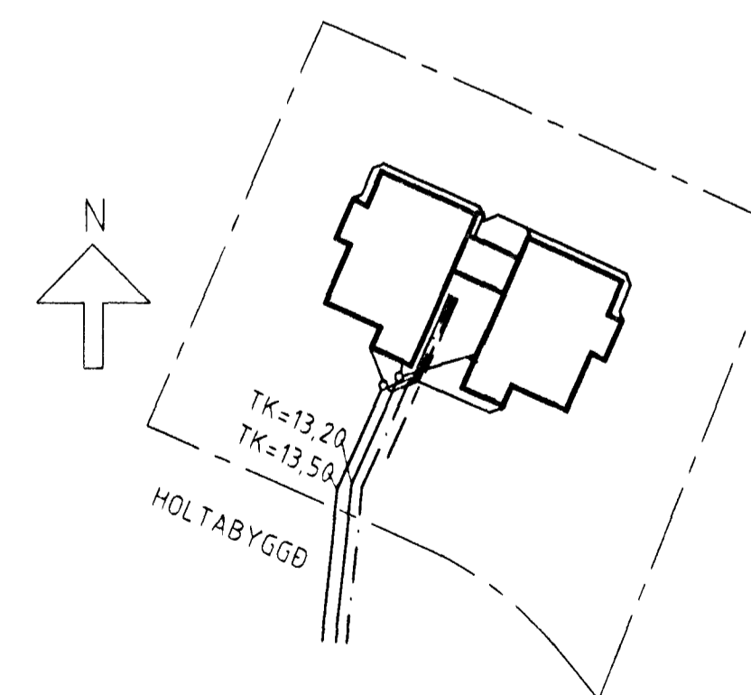
AFSTÖÐUMYND M, 1:500
