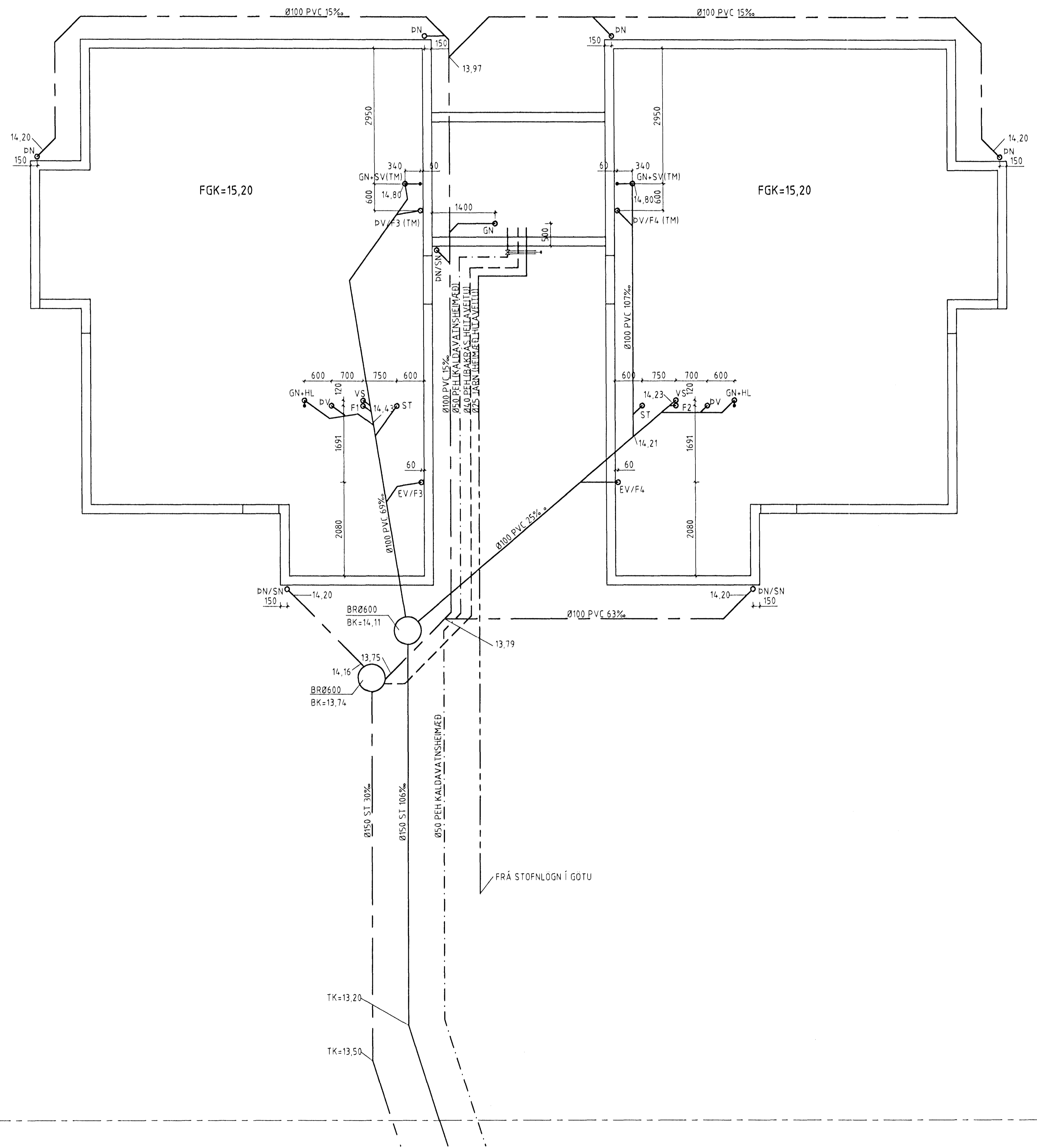
AFSTÖÐUMYND M, 1:500
