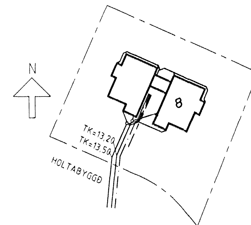
AFSTÖÐUMYND M, 1:500
