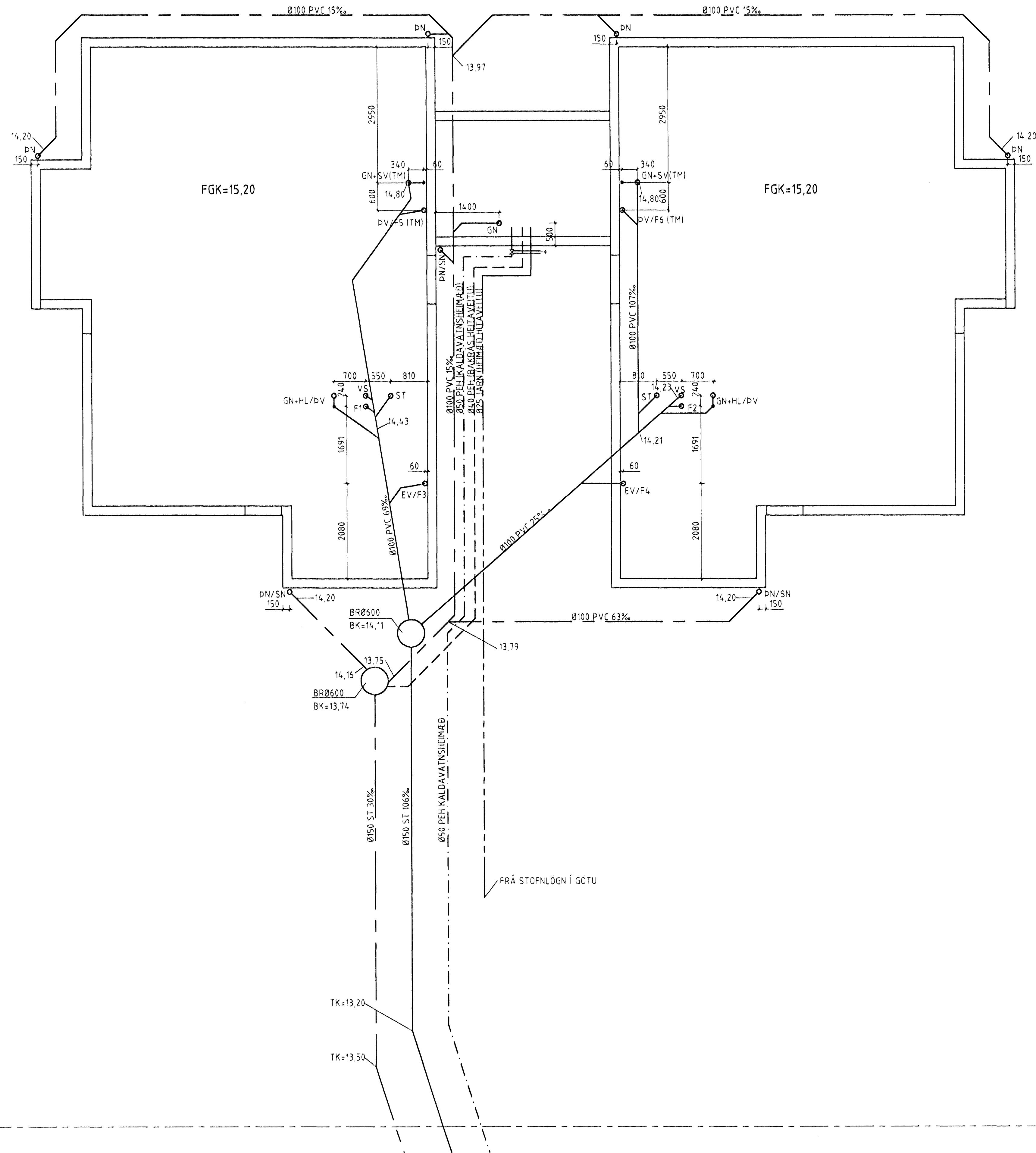
AFSTÖÐUMYND M, 1:500
