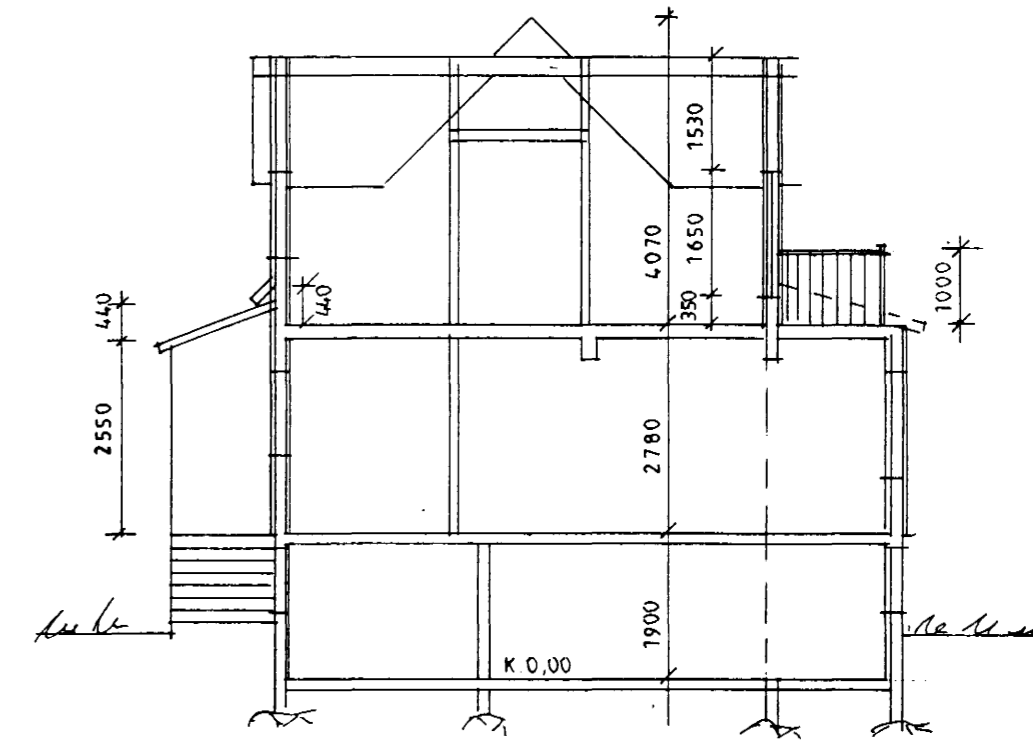
SNÍÐ A-A
