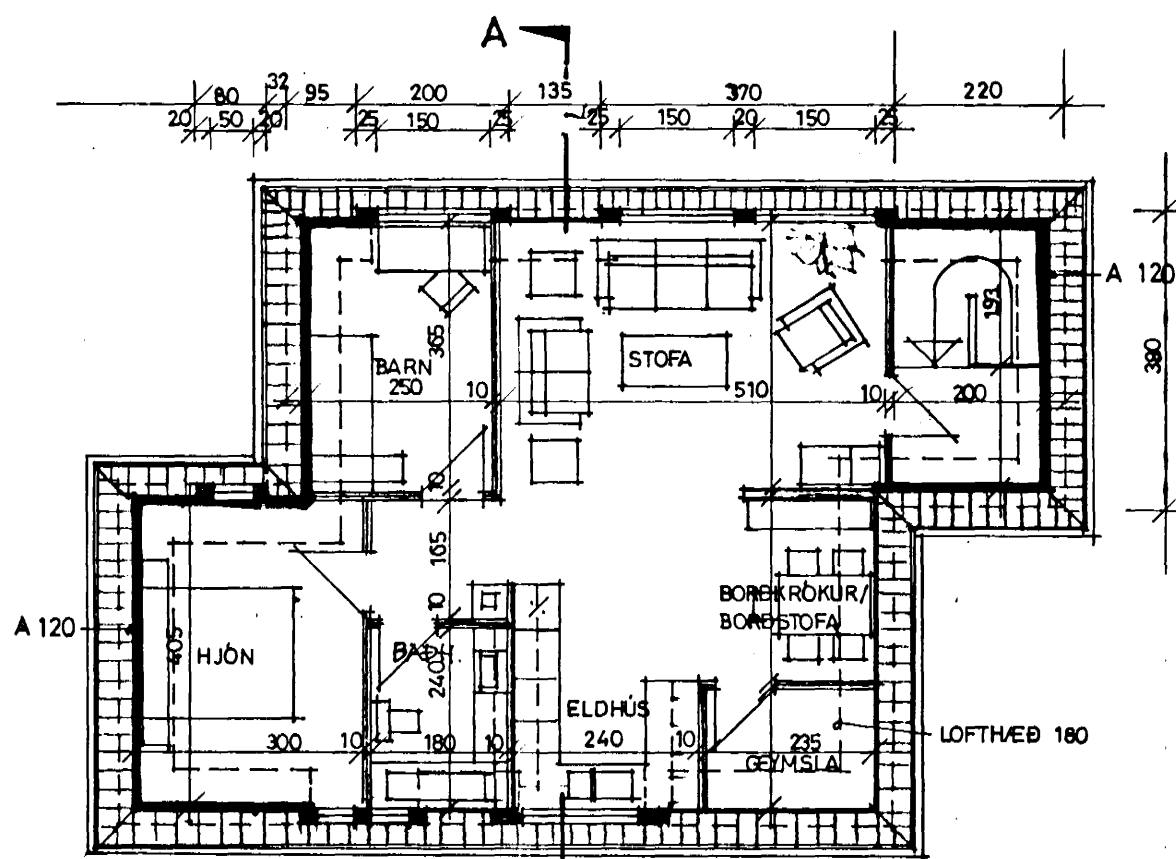
RISHÆÐ
