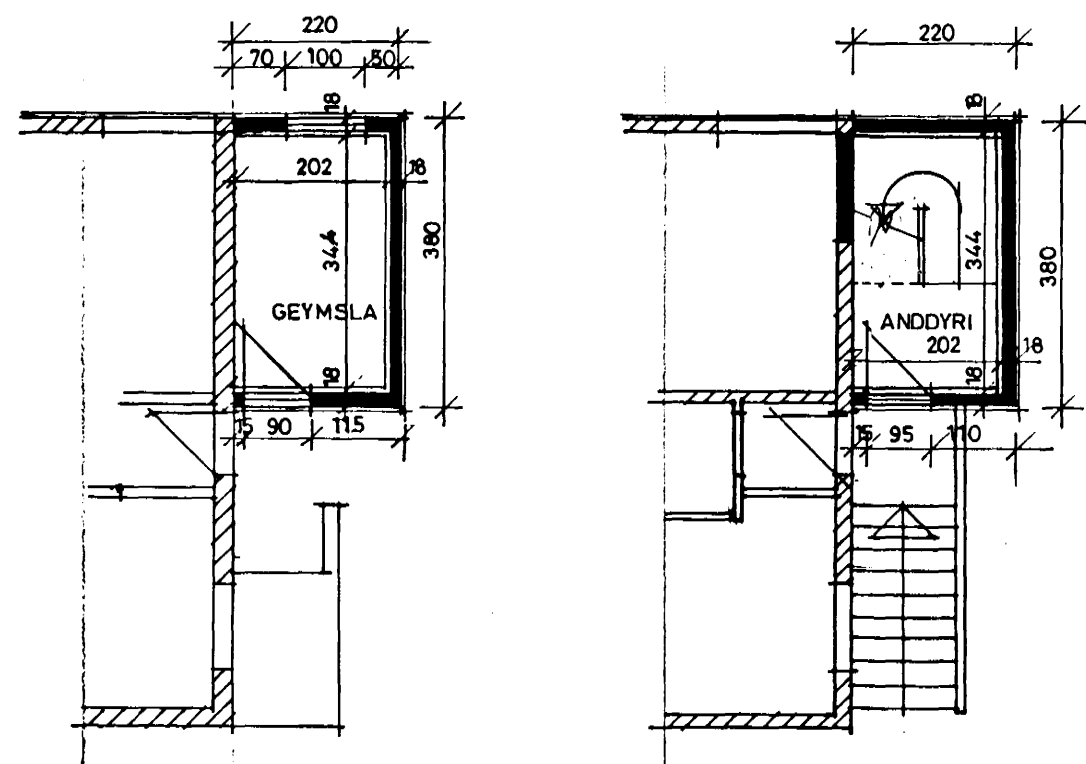
KJALLARI
