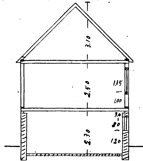
Skurður.
