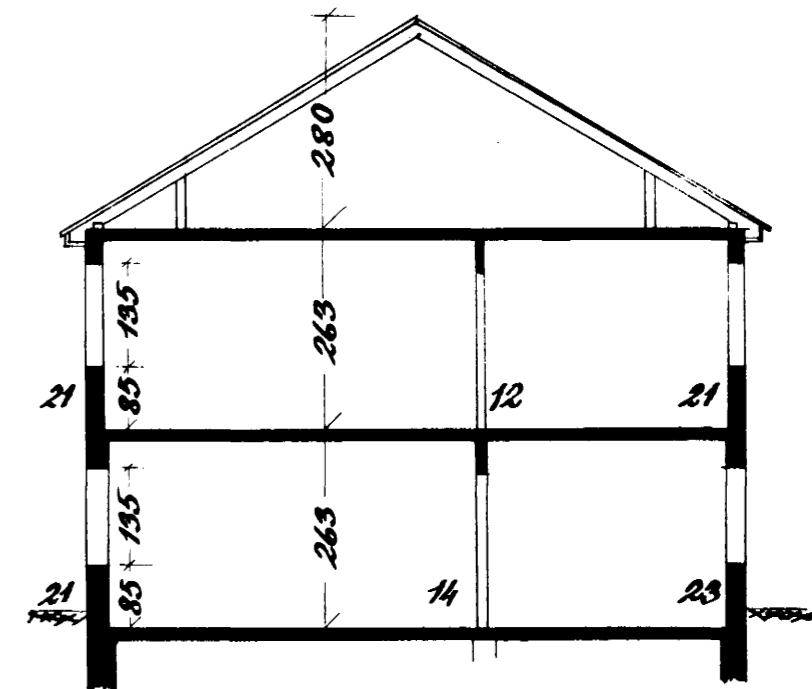
Þverskurður
