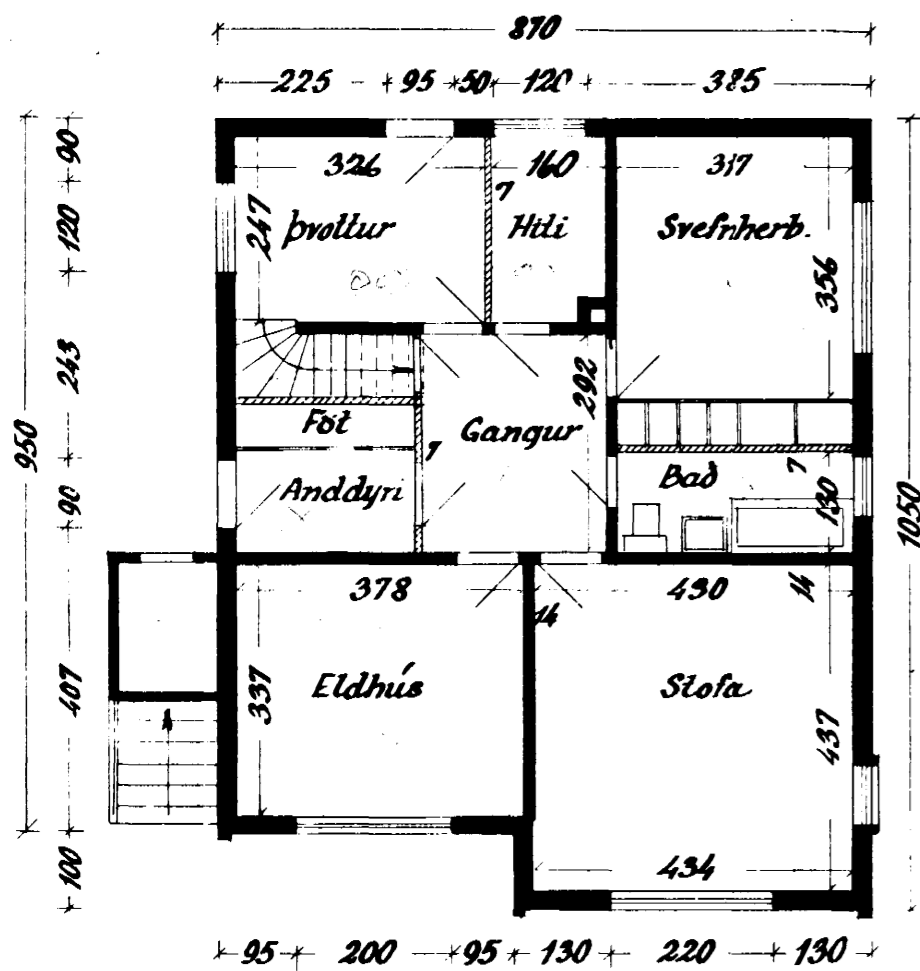
1. hæð
