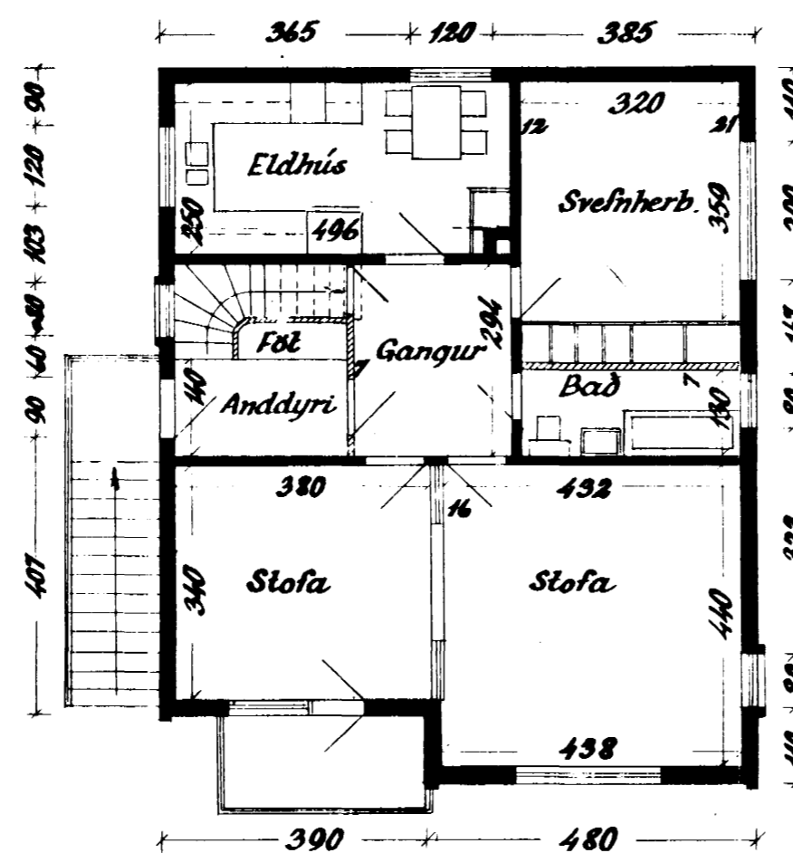
2. hæð
