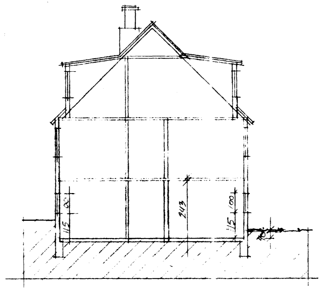
SNIÐ 1:100
