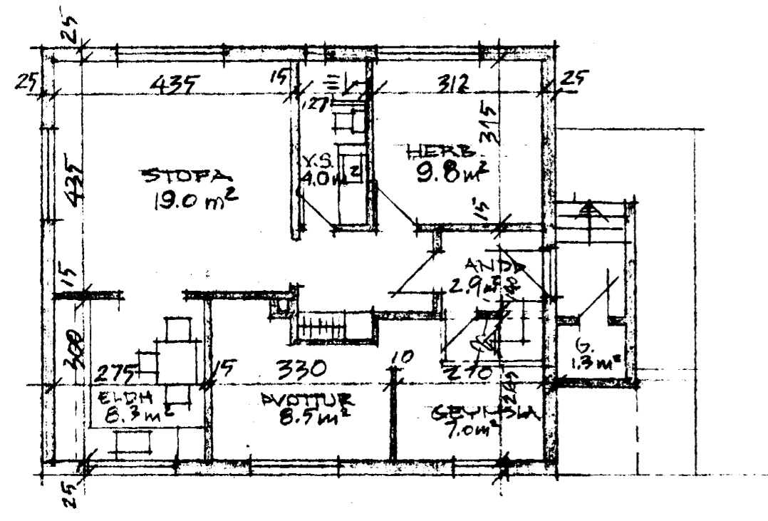
GRUNNMYND JARDHÆÐAR 1:100
