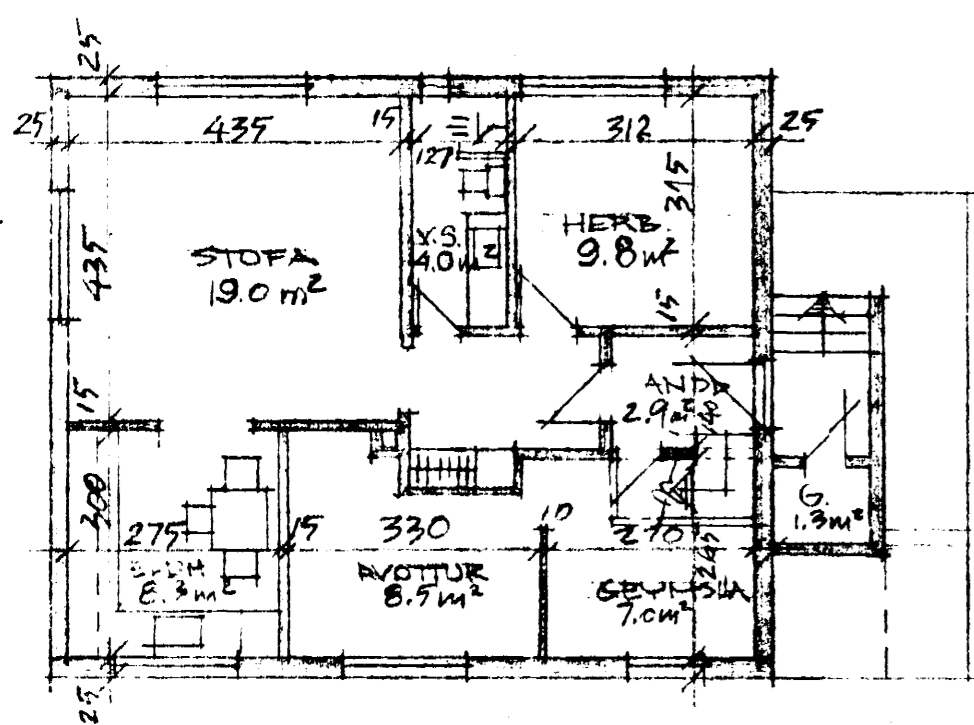
GRUNNMYND JARÐHÆÐAR 1:100
