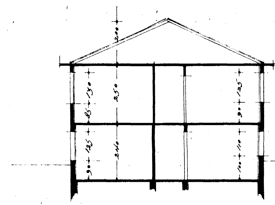
Skurður A-A
