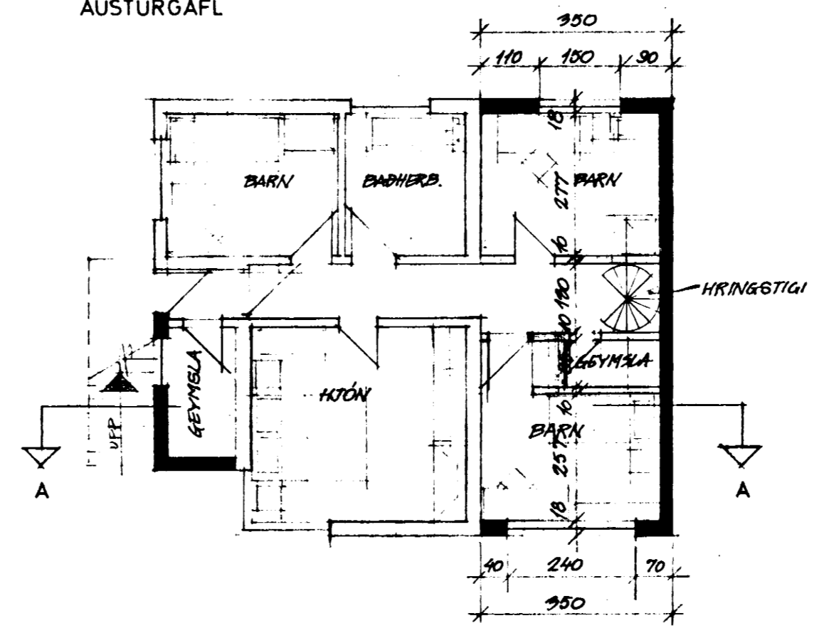
GRUNNMYND JARÐHÆÐAR
