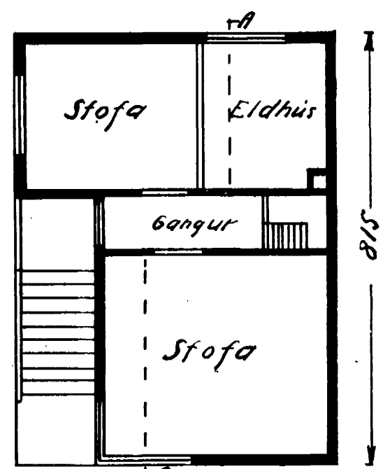
1 Hæð.
