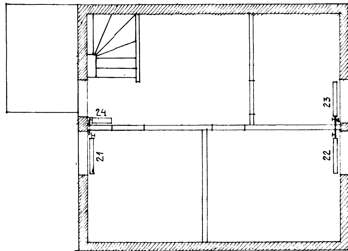
2. HÆÐ. 1:50.
