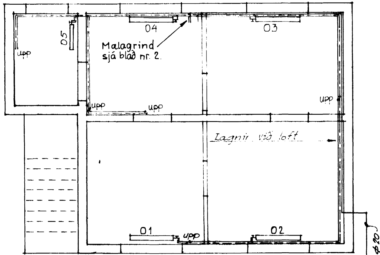
KJALLARI. 1:50.
