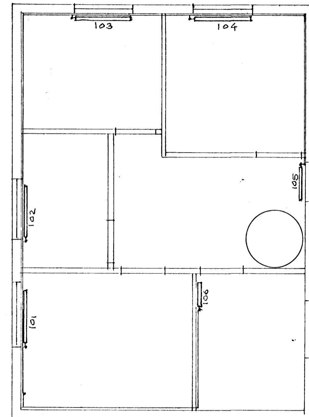
1. HÆÐ 1:50
