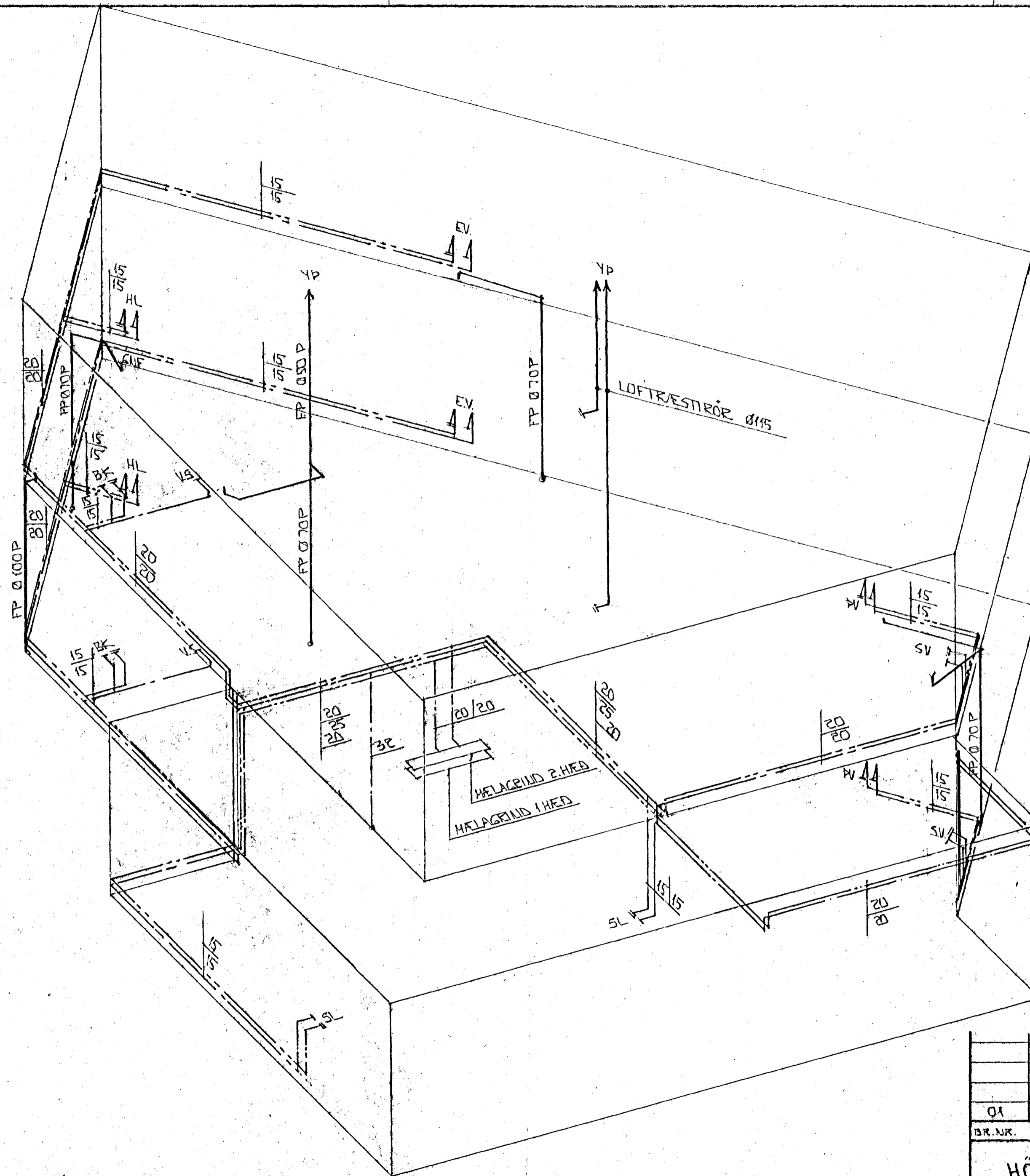
RÚMMYND 1:50
