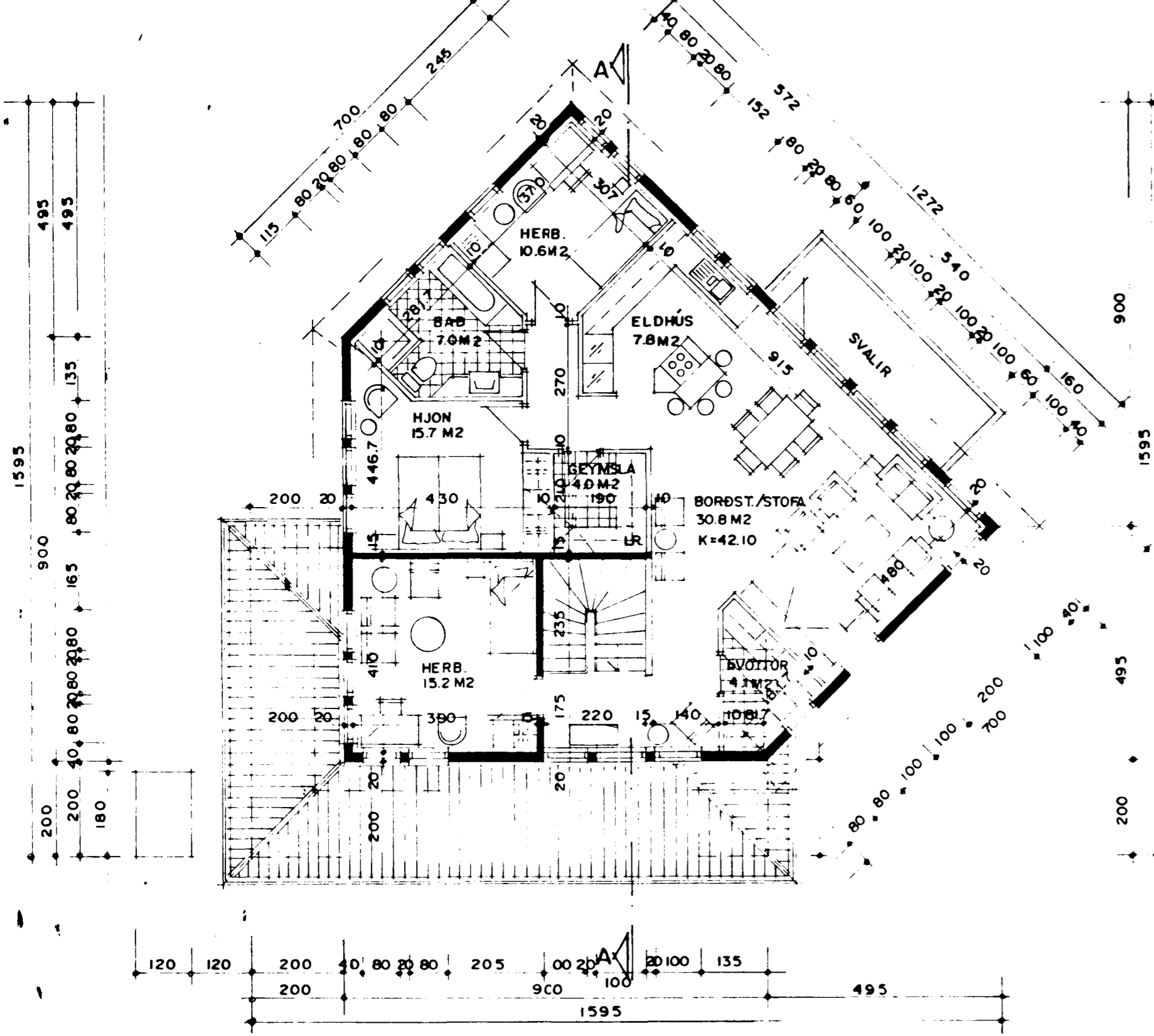
VESTURHLIÐ MKV. 1:100
