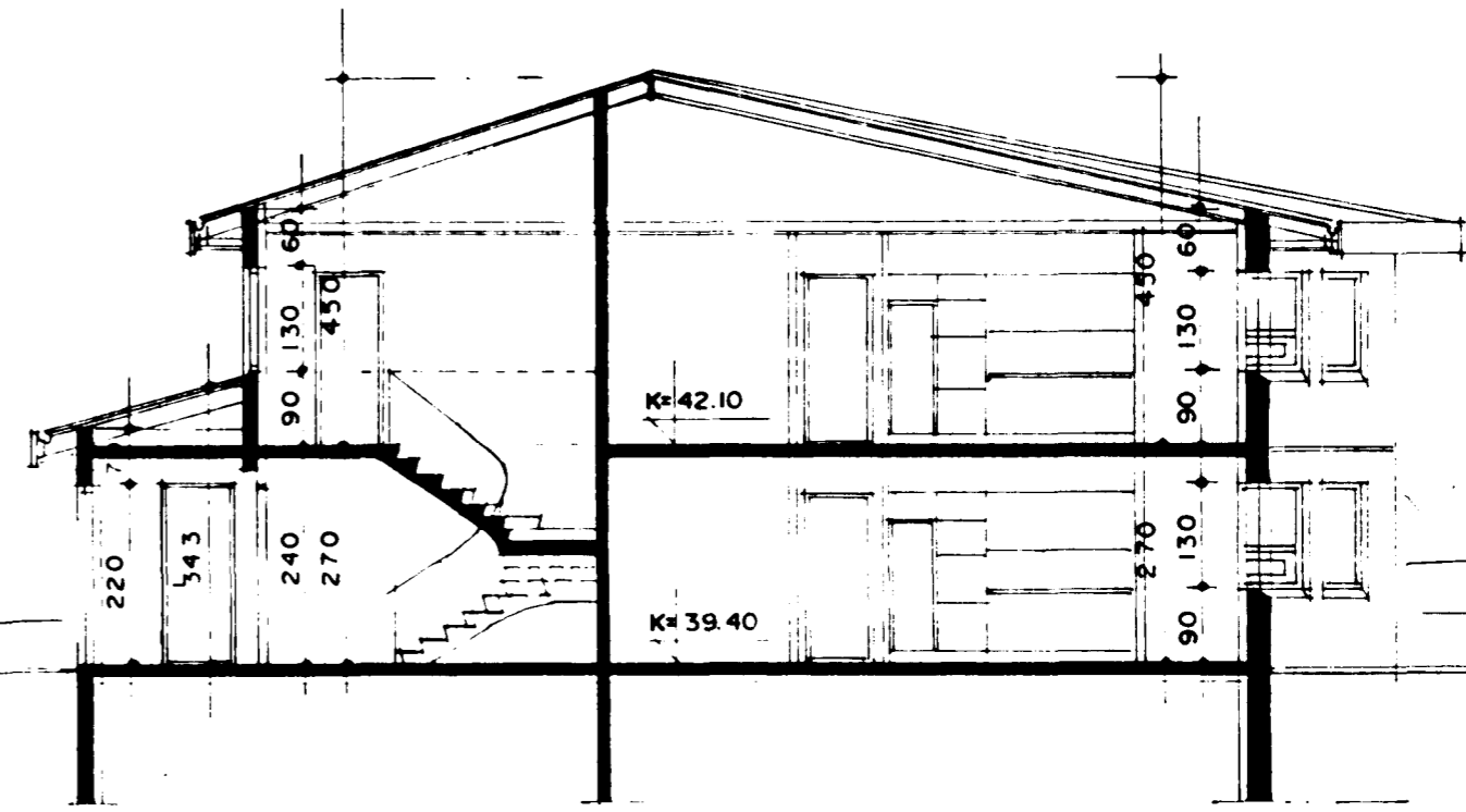
SNEIÐING A-A MKV. 1:100
